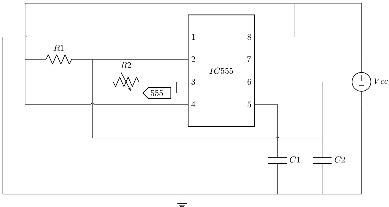
Figura 24: Circuito oscilador astable.
