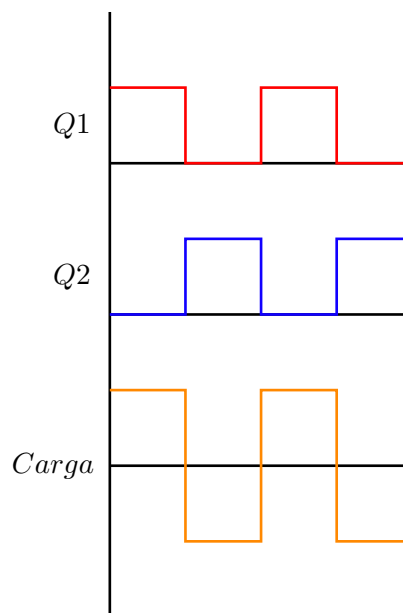
Figura 28: Forma de onda.
