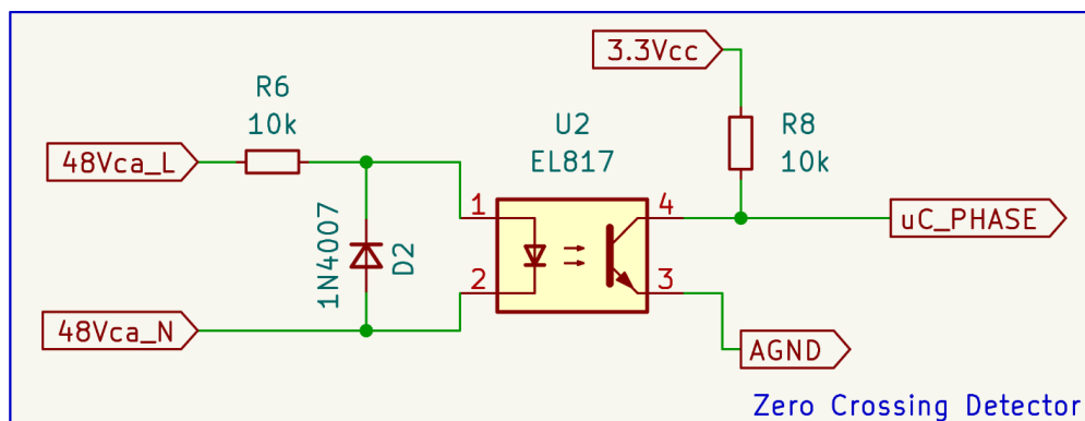
Figura 19: Circuito detector de cruce por zero utilizado.
