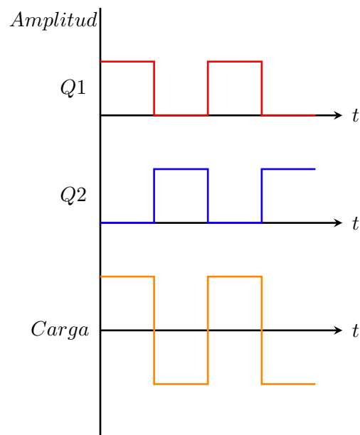
Figura 27: Forma de onda.
