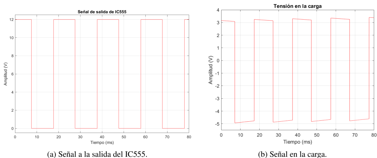
Figura 30: Gráficos de simulación
