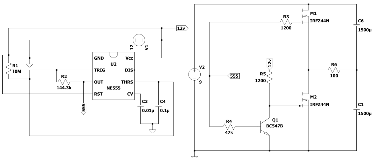
Figura 29: Circuito en LTSpice.
