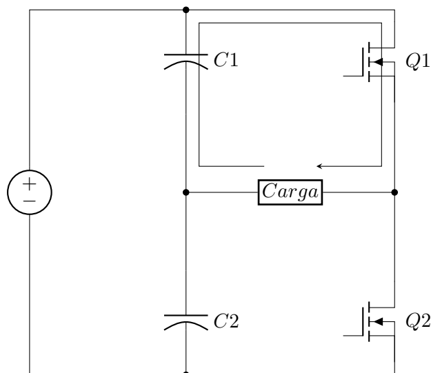
Figura 25: Conmutación 1.
