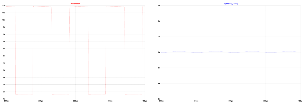
(a) Tensión en drenador de transistor de conmutación.
