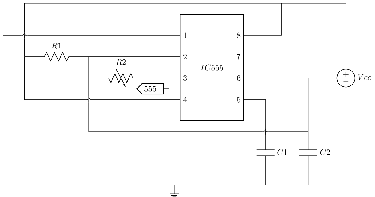
Figura 23: Circuito oscilador astable.
