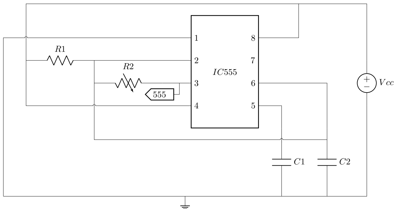
Figura 26: Circuito oscilador astable.
