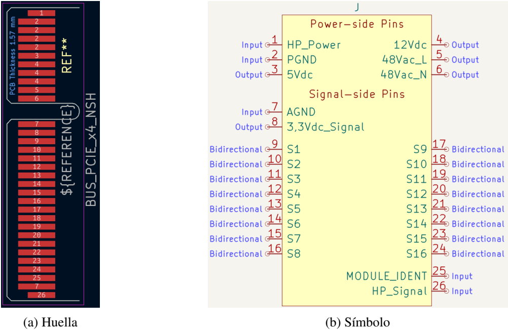
Figura 33: Símbolo y huella del conector PCIe x4
