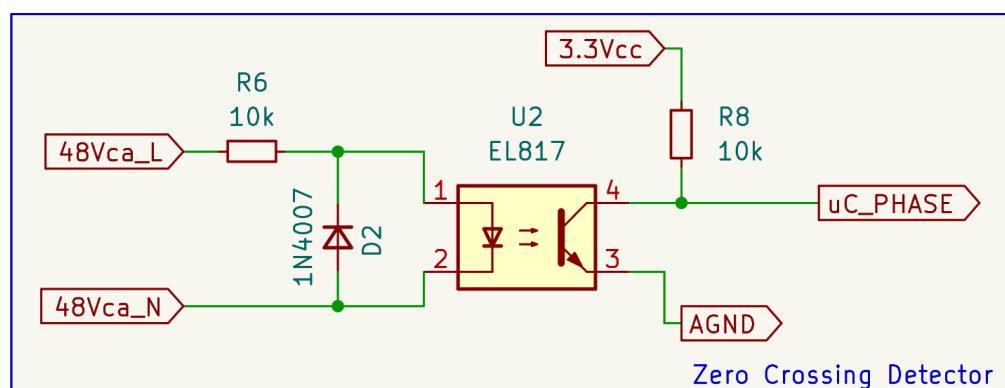
Figura 19: Circuito detector de cruce por cero utilizado.
