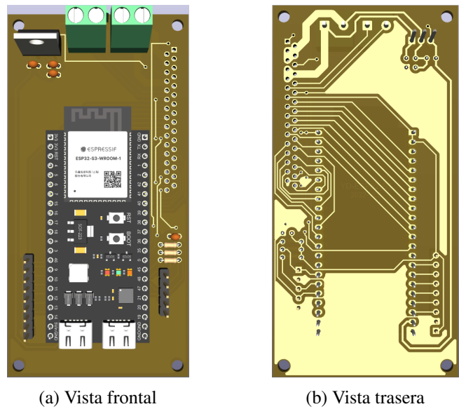
Figura 35: Modelo 3D de las PCB general del control del gabinete.
