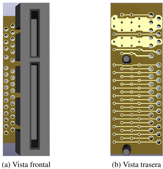
Figura 36: Modelo 3D de la mini-PCB para el conector PCIe x4.
