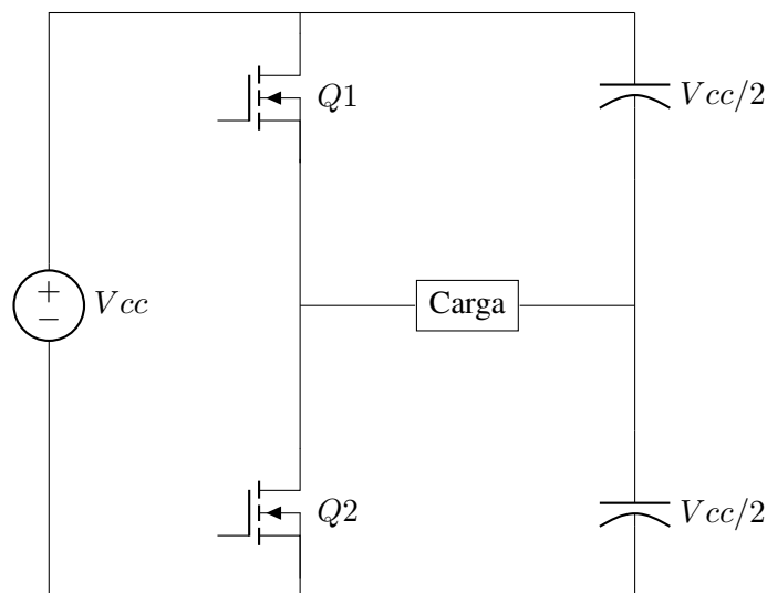
Figura 31: Inversor medio puente con control por 555
