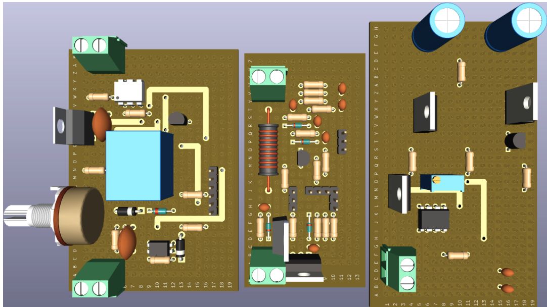
Figura 32: Vista frontal de los modelos 3D de las placas experimentales perforadas. De izquierda a derecha: módulo recortador de onda, módulo convertidor Buck, módulo inversor de onda cuadrada
