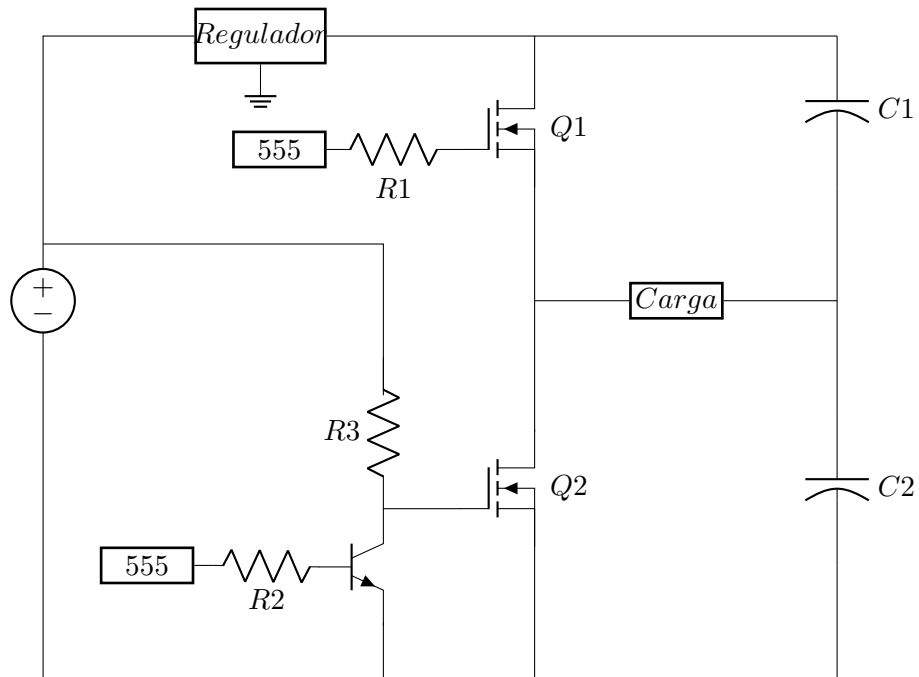
Figura 27: Circuito de inversor medio puente.
