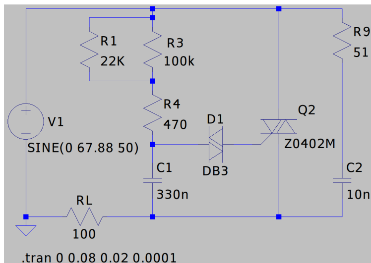
Figura 23: Circuito en LTSpice 2
