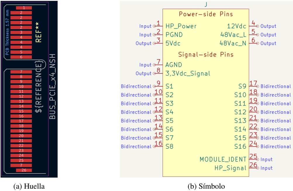
Figura 30: Símbolo y huella del conector PCIe X4
