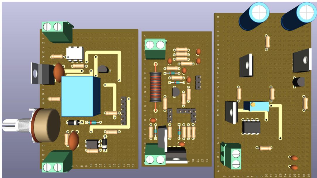
Figura 29: Vista frontal de los modelos 3D de las placas experimentales perforadas. De izquierda a derecha: módulo recortador de onda, módulo convertidor Buck, módulo inversor de onda cuadrada
