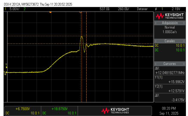
(b) Con capacitor de 2 pF 1 .
