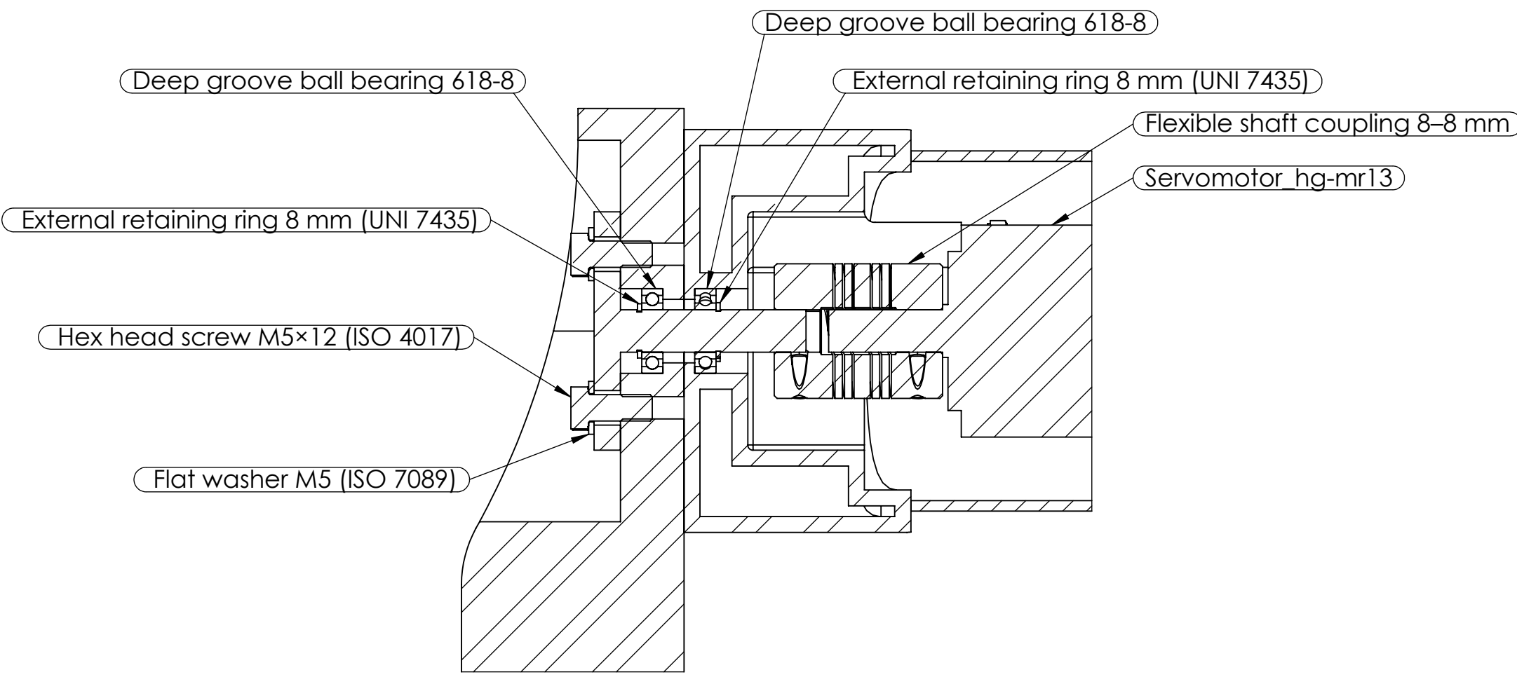
SECTION A-A SCALE 1 : 1
