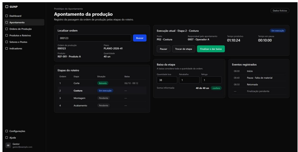
Figura 7 – Protótipo da Tela de Apontamento da Produção
