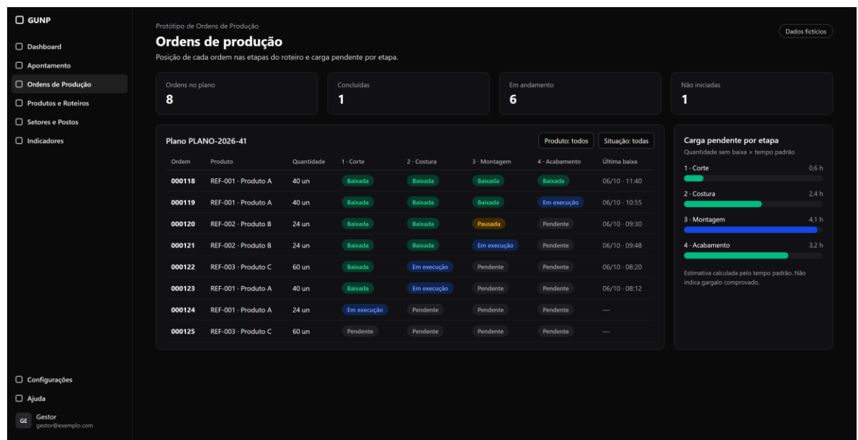
Figura 8 – Protótipo da Tela de Ordens de Produção
