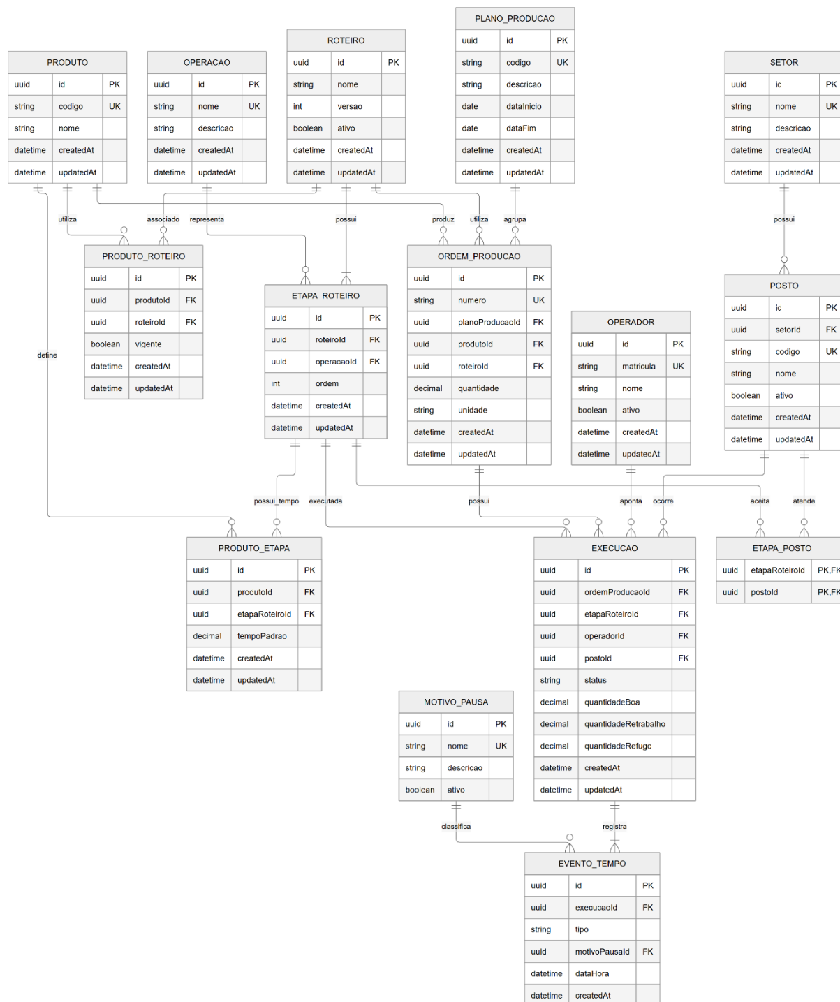
Figura 9 – Diagrama Entidade-Relacionamento do Banco de Dados
