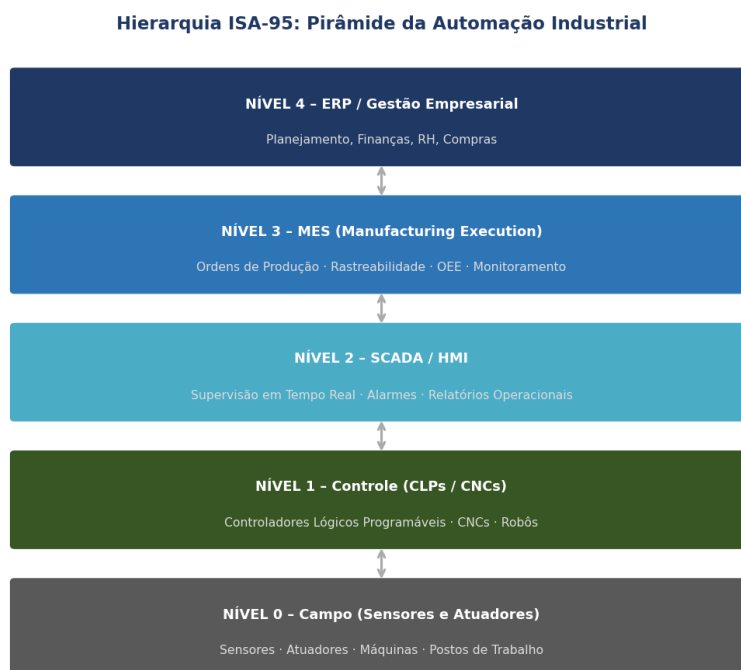
Figura 3 – Hierarquia ISA-95: Pirâmide da Automação Industrial
