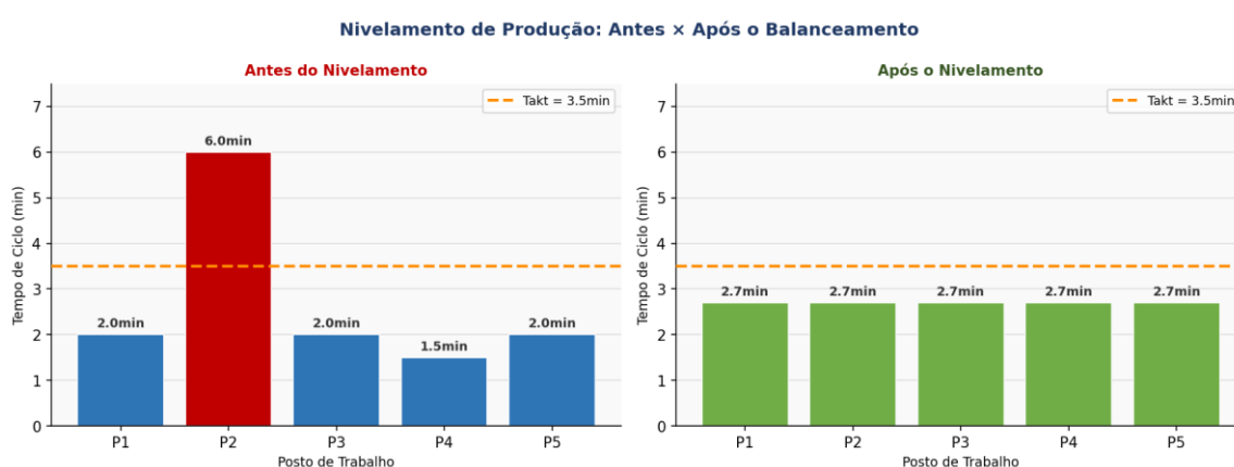
Figura 2 – Nivelamento de Produção: Antes e Após o Balanceamento das Atividades
