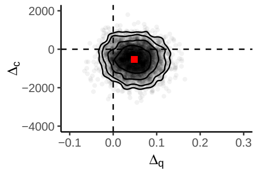
suBART
