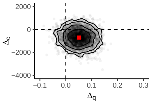
ps-mvBART
