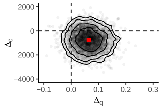
ps-suBART
