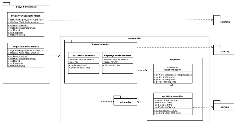
Abbildung 3.3: Klassendiagramm
