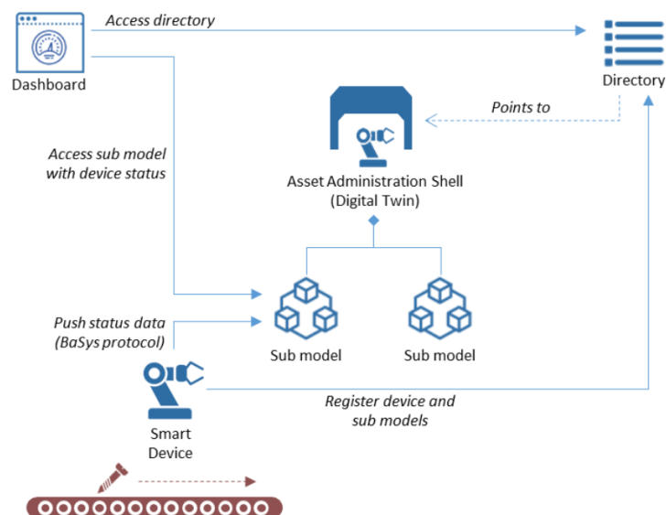
Abbildung 2.2: Beispiel einer einfachen BaSys-Architektur ([4])
