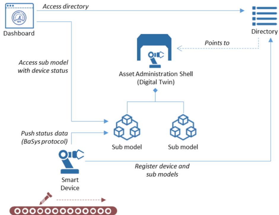
Abbildung 2.6: Beispiel einer BaSys-Architektur [2]
