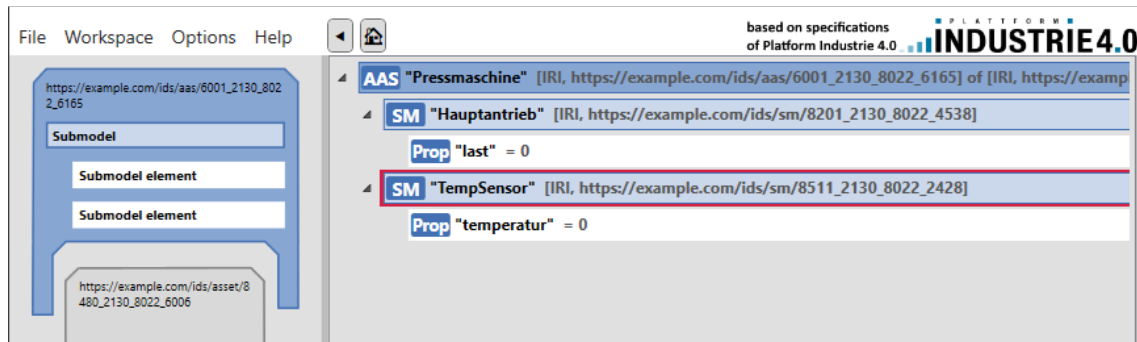
Abbildung 4.4: Bildschirmaufnahme der Verwaltungsschale auf AASXExplorer
