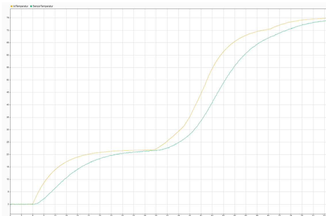
Abbildung 4.2: Verläufe von dem Augenblickswert und dem vom Sensor abgetasteten Wert der Temperatur an der Kontaktstelle
