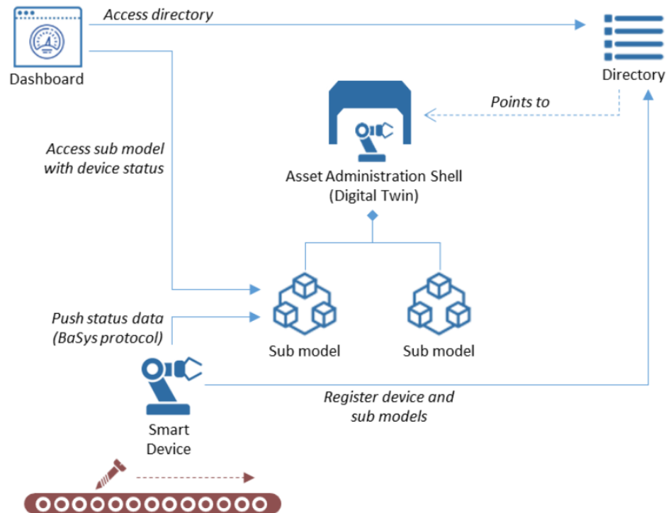
Abbildung 2.7: Beispiel einer BaSys-Architektur [2]
