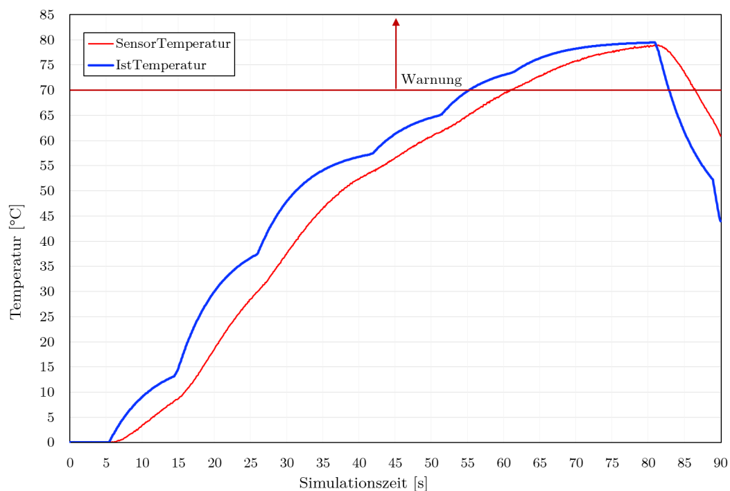
Abbildung 4.3: Verläufe des Ist-Wertes und des vom Sensor abgetasteten Wertes der Temperatur an der Kontaktstelle
