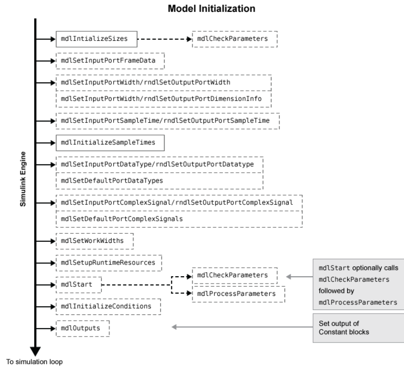
Abbildung 2.4: Ablaufreihenfolge, wenn das Modell initialisiert ist [12]
