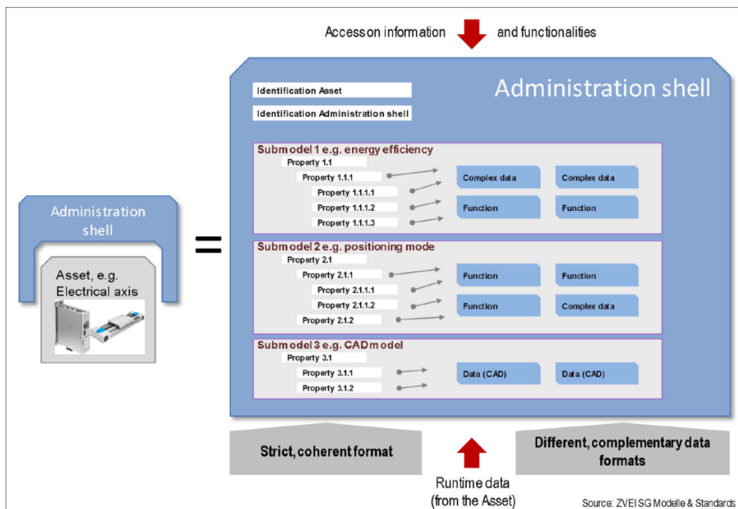
Abbildung 2.4: Abbild eines AAS [2]
