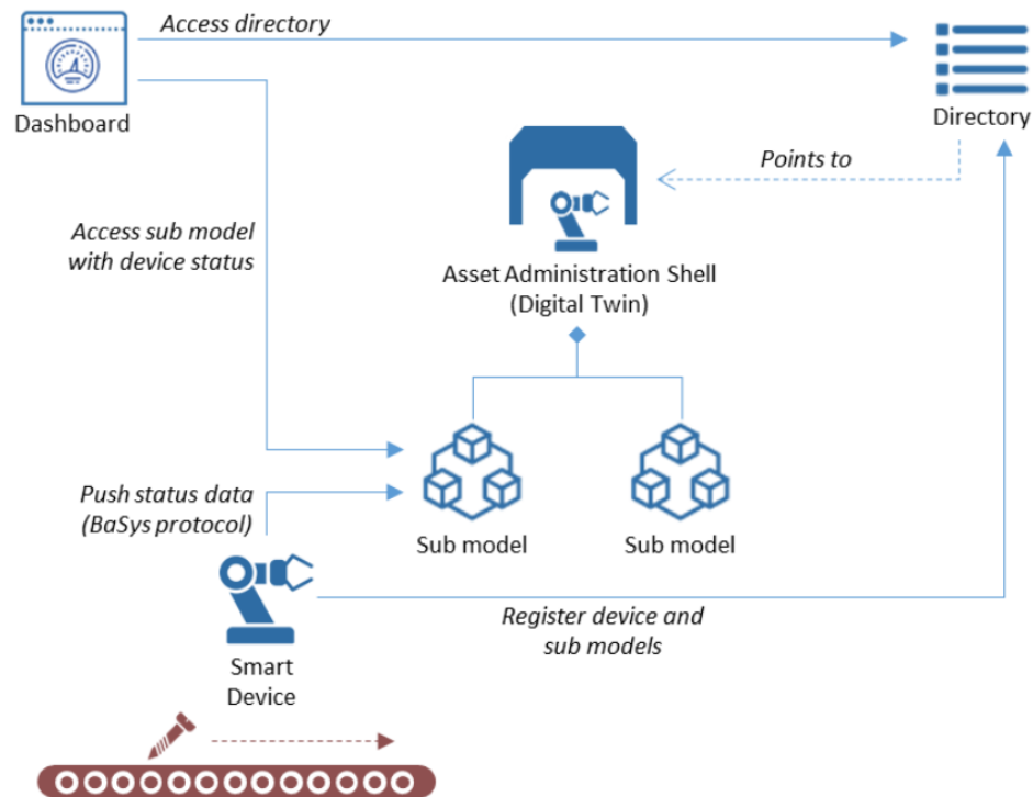
Abbildung 2.3: Beispiel einer einfachen BaSys-Architektur [2]
