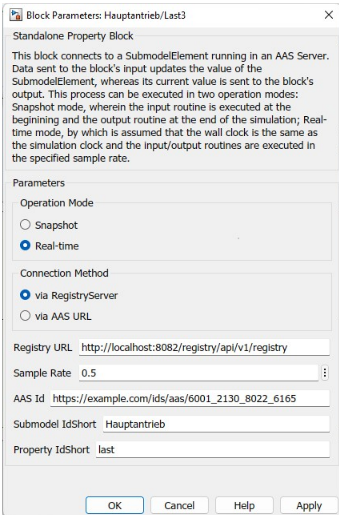
Abbildung 3.10: Dialogfenster des PropertySACconnector-Block
