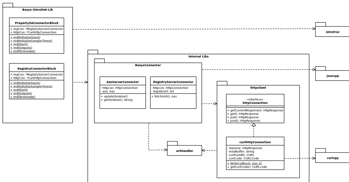
Abbildung 3.3: Klassendiagramm
