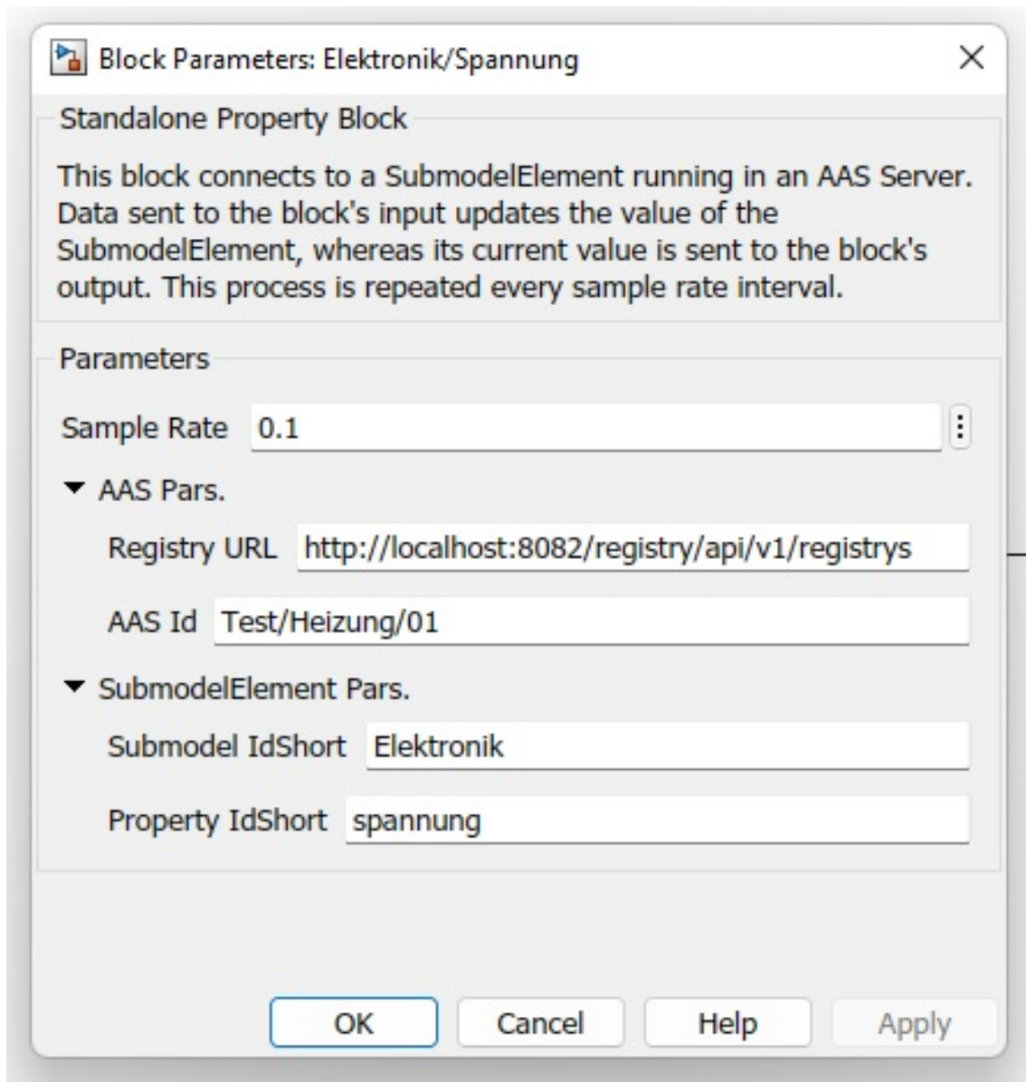
Abbildung 3.10: Dialogfenster des PropertySACconnector-Block
