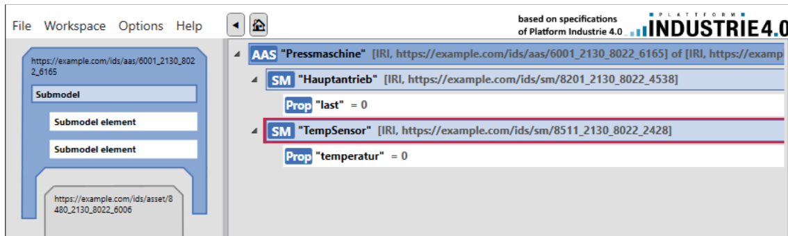
Abbildung 4.1: Bildschirmaufnahme der Verwaltungsschale auf AASXExplorer
