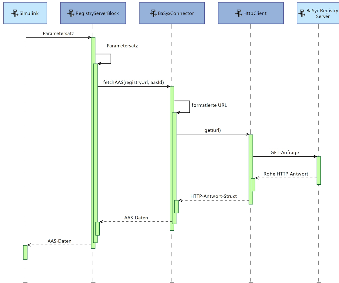
Abbildung 3.6: Sequenzdiagramm für A3
