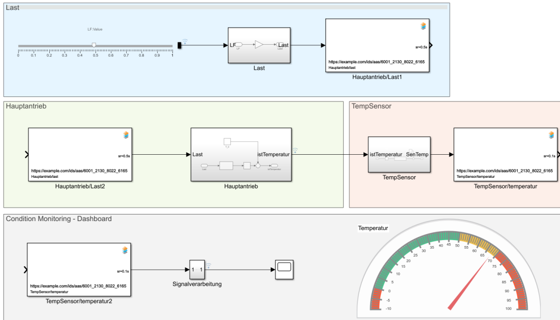
Abbildung 4.2: Simulink-Modell des Beispielszenarios
