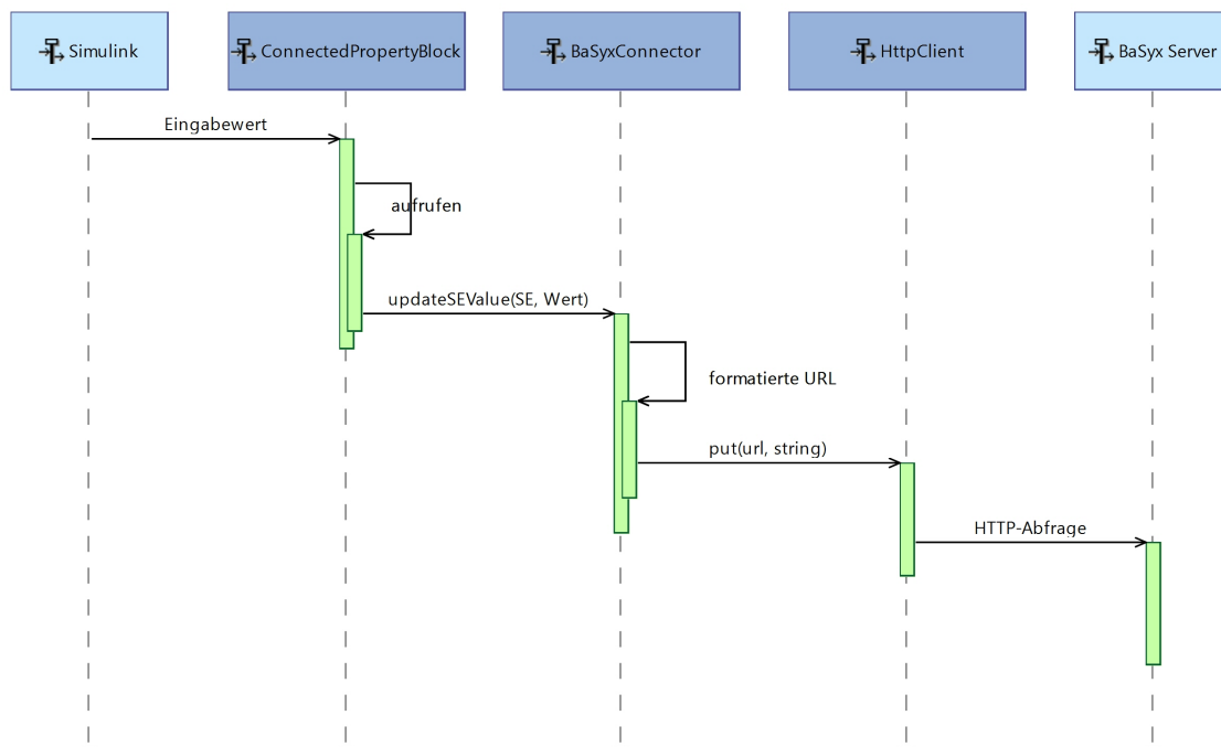
Abbildung 3.5: Sequenzdiagramm für A2
