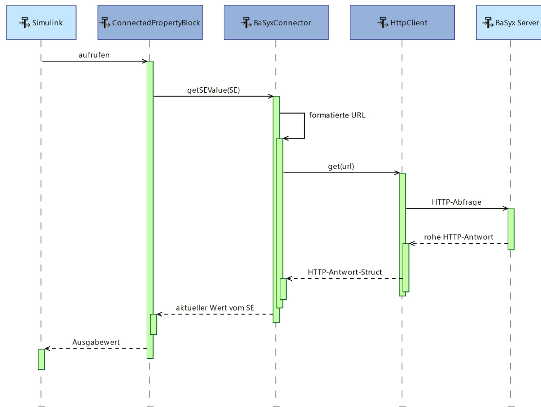
Abbildung 3.4: Sequenzdiagramm für A1
