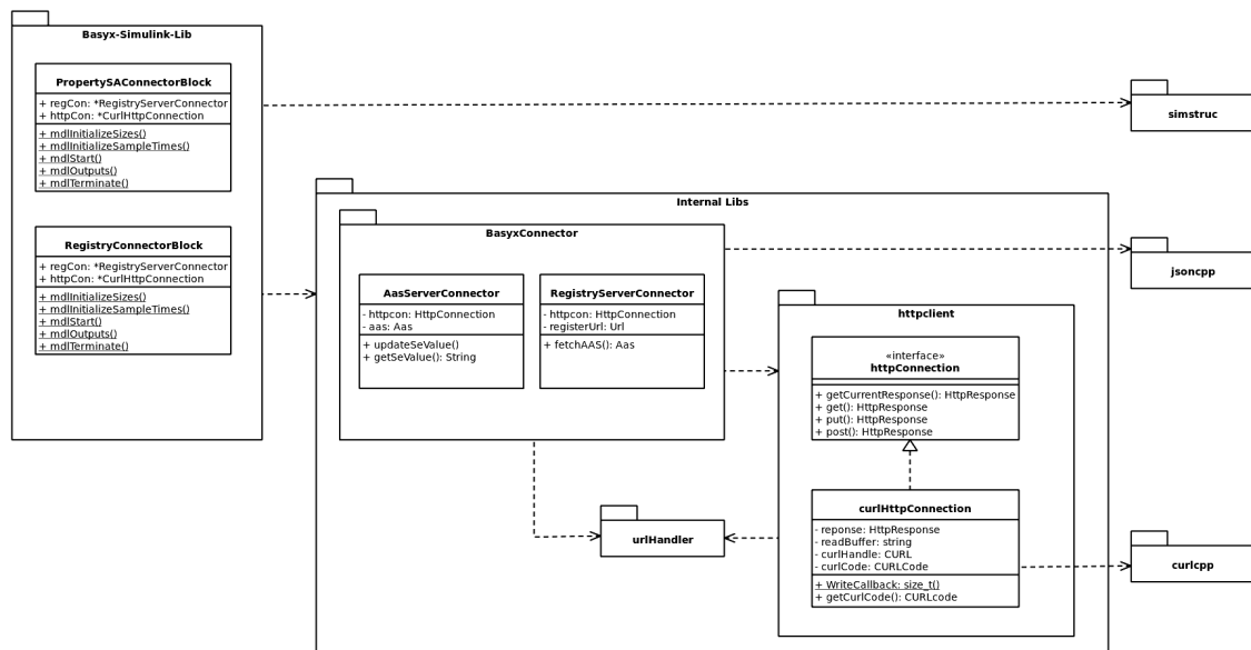
Abbildung 3.3: Klassendiagramm
