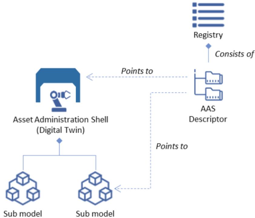
Abbildung 2.10: Diagramm einer Eclipse BaSys-Systemstruktur [2]
