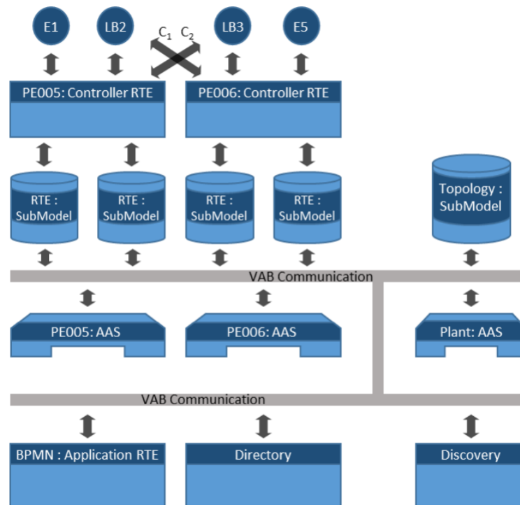
Abbildung 2.5: VAB-Beispiel mit verbundenen Entitäten [2]
