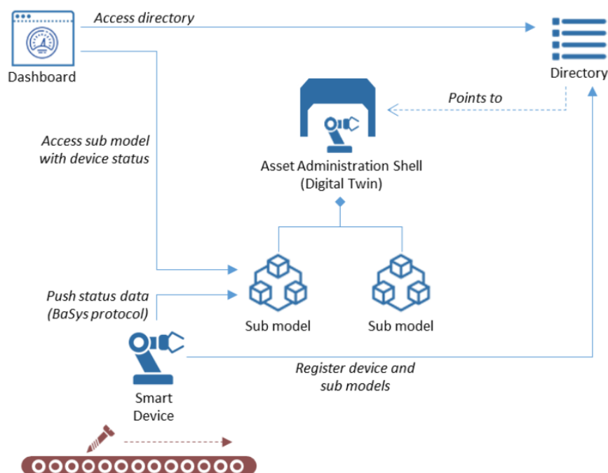
Abbildung 2.3: Beispiel einer einfachen BaSys-Architektur [2]
