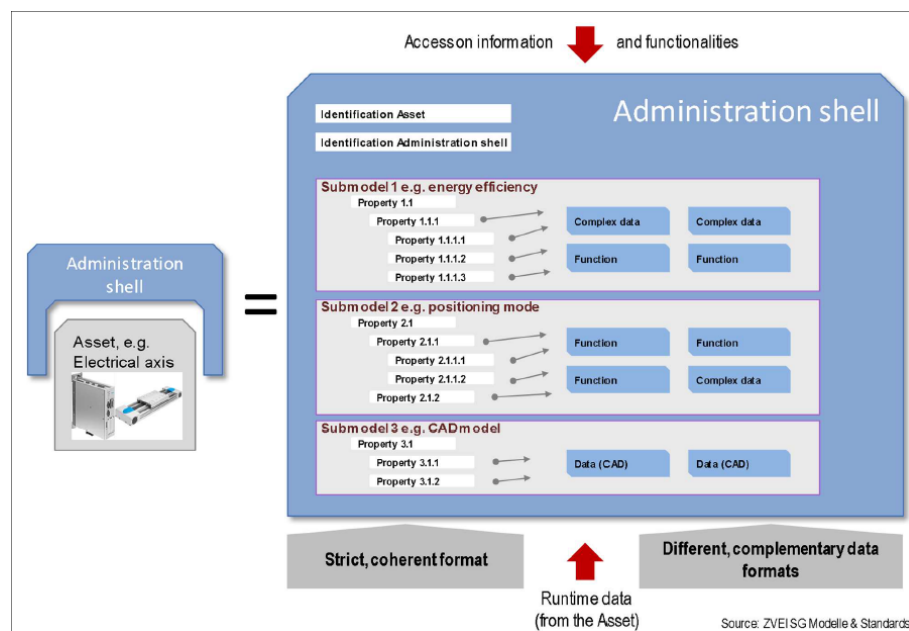
Abbildung 2.4: Abbild eines AAS [2]
