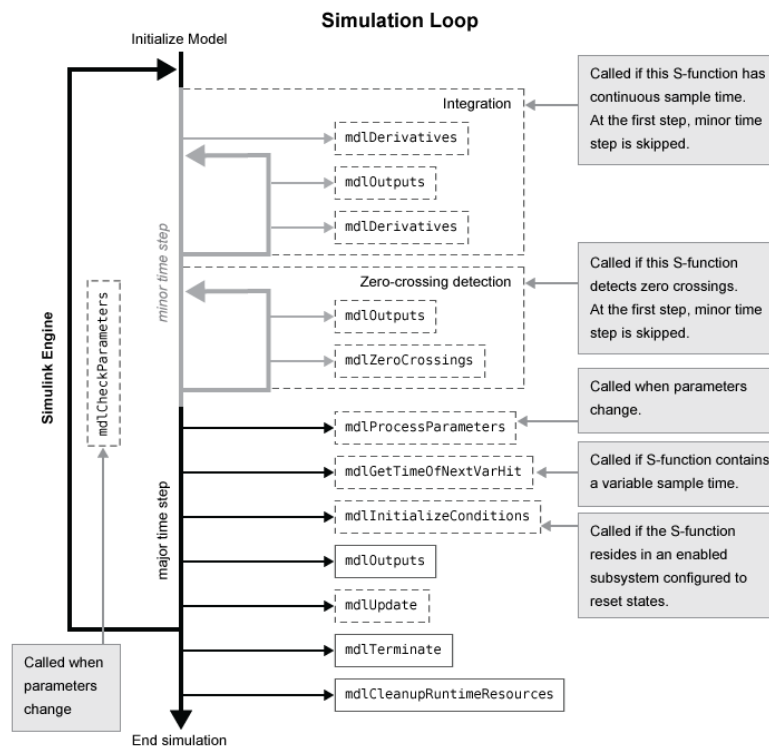
Abbildung 2.4: Simulationsschleife einer mit C MEX erstellten S-function [11]
