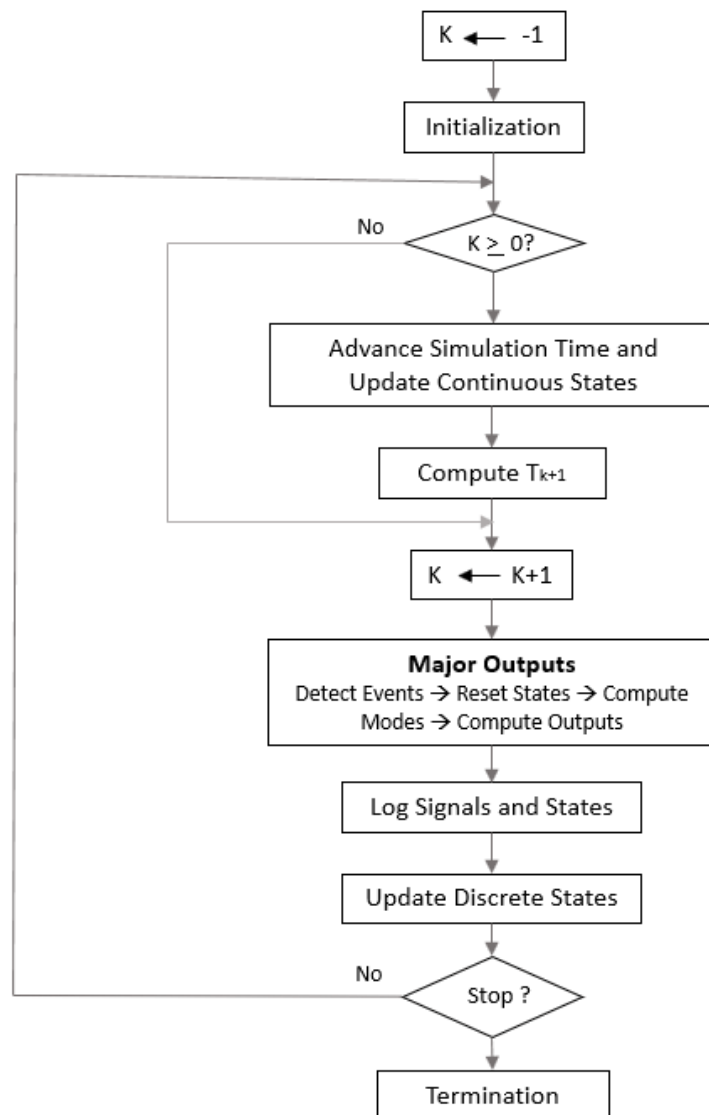
Abbildung 2.2: Struktur eines Simulationssdurchlaufes in Simulink, wobei k als Zähler für den Major -Zeitschritt dient
