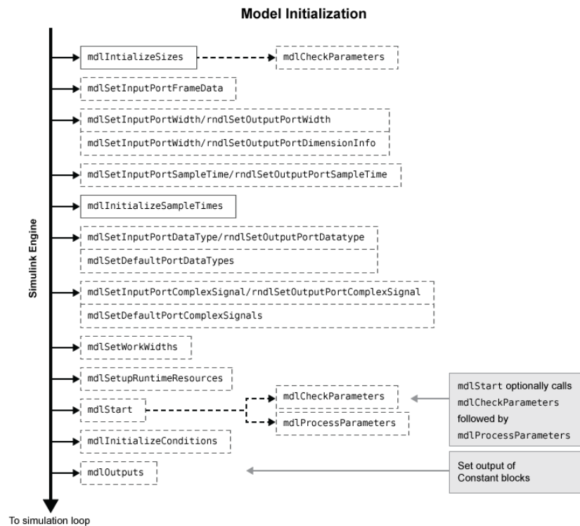
Abbildung 2.3: Ablaufreihenfolge, wenn das Modell initialisiert ist [11]
