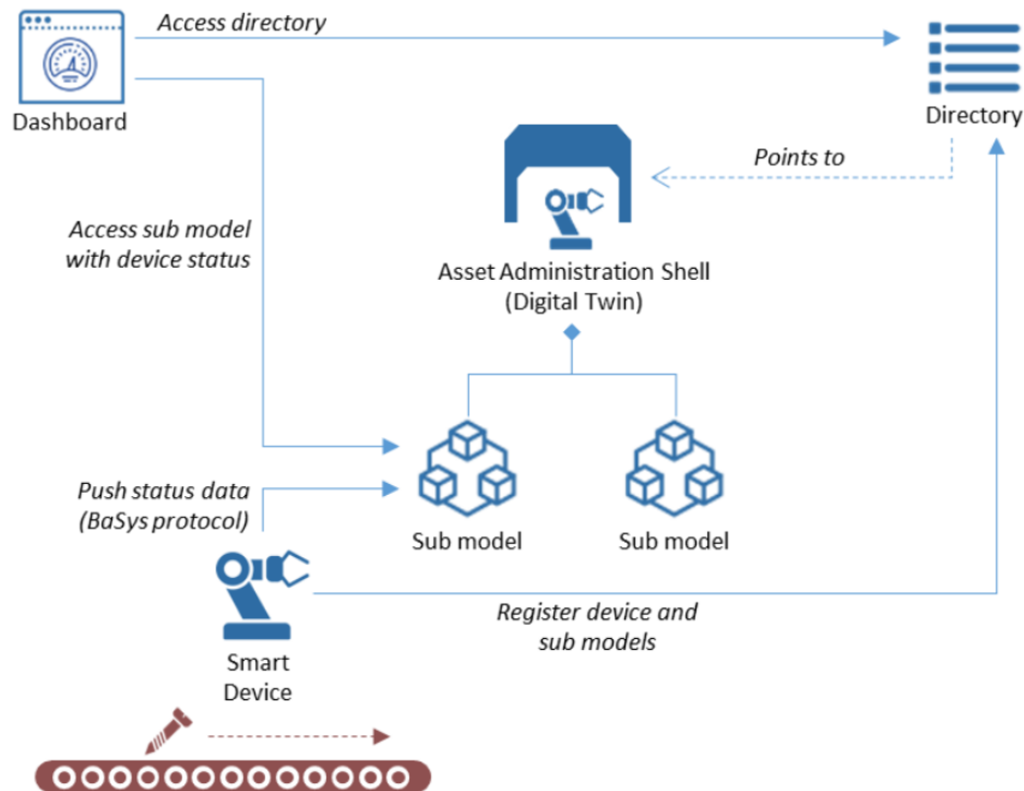
Abbildung 2.6: Beispiel einer einfachen BaSys-Architektur [2]
