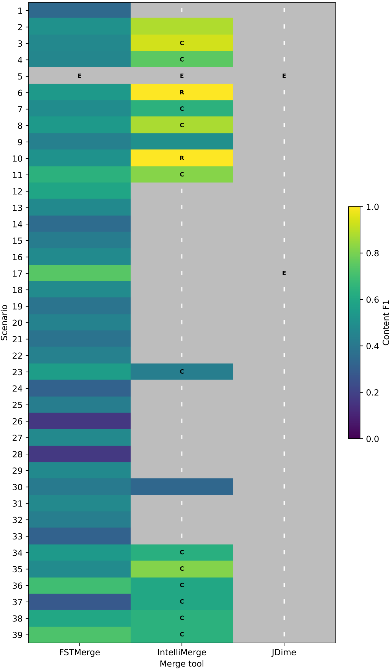
Scenario-level content F1 and terminal outcome
