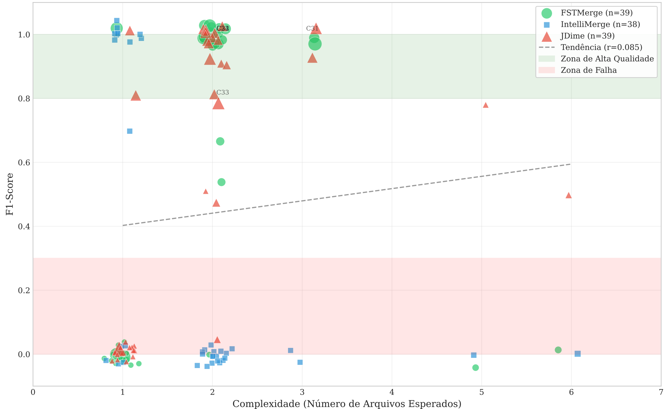
Relação entre Complexidade do Cenário e Qualidade do Merge
