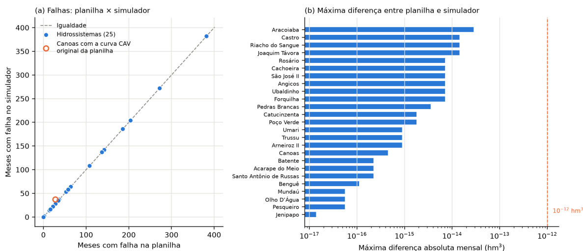
Figura 7 – Verificação numérica nos 25 hidrossistemas: (a) meses com falha na planilha e no simulador; (b) máxima diferença absoluta mensal entre os dois cálculos.
