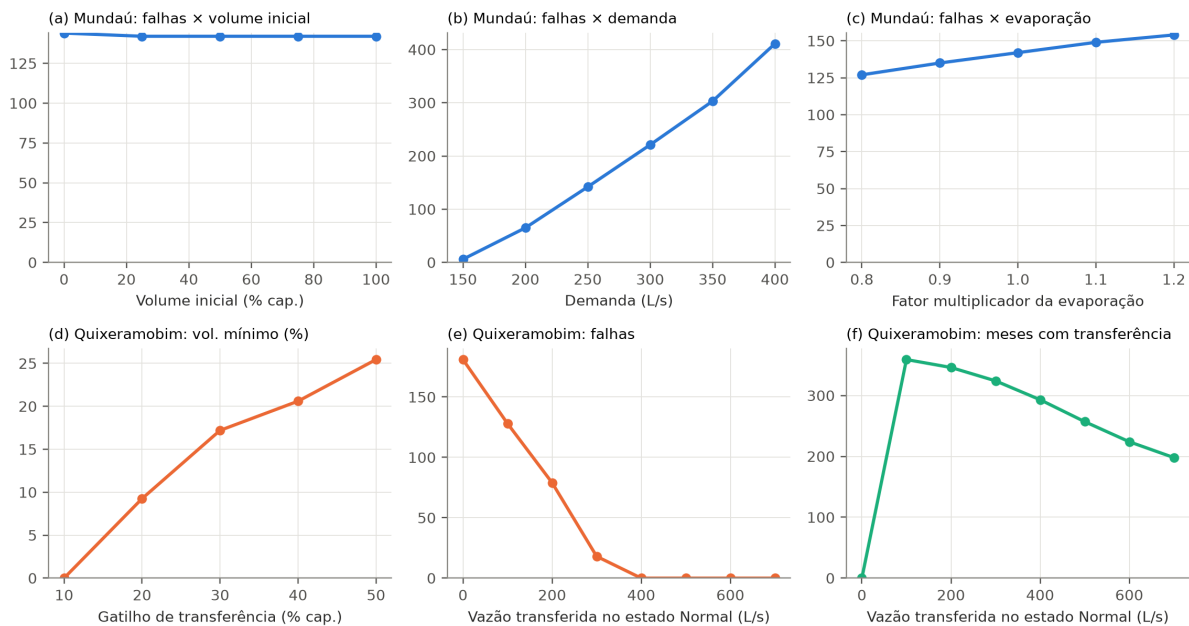
Figura 8 – Sensibilidade dos indicadores ao volume inicial, à demanda e à evaporação (Mundaú) e ao gatilho e à vazão de transferência (Fogareiro–Quixeramobim).
