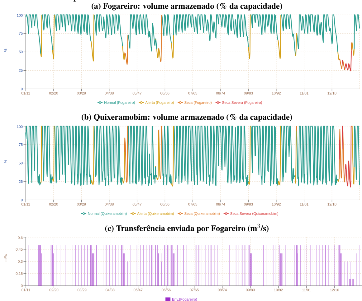
Figura 15 – Resultados de Fogareiro–Quixeramobim exportados pelo simulador (1911–2019): volumes coloridos pelo estado do sistema e vazão transferida.
