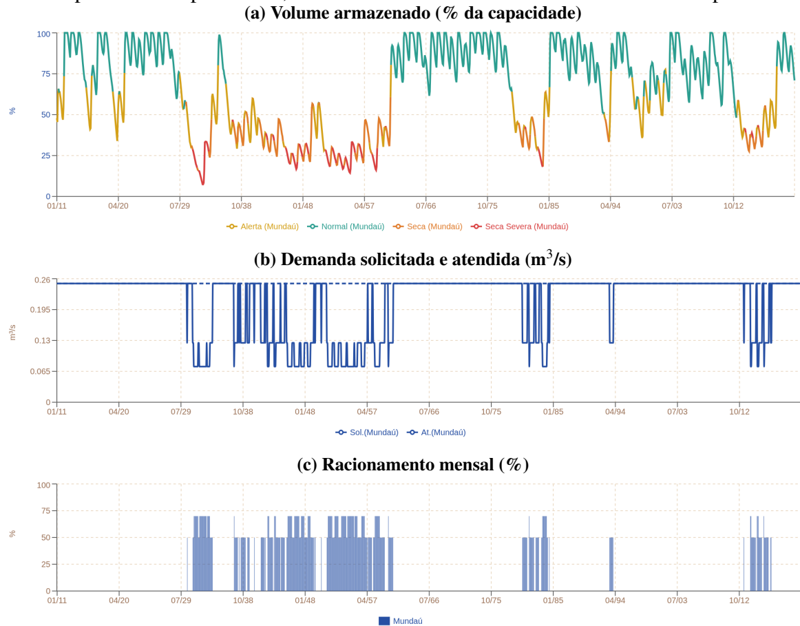
Figura 9 – Resultados de Mundaú exportados pelo simulador (1911–2021): volume armazenado colorido pelo estado operacional, demanda solicitada e atendida e racionamento aplicado.
