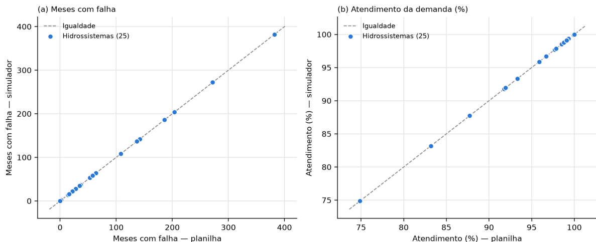
Figura 7 – Verificação numérica nos 25 hidrossistemas: (a) meses com falha e (b) atendimento da demanda calculados pela planilha e pelo simulador.
