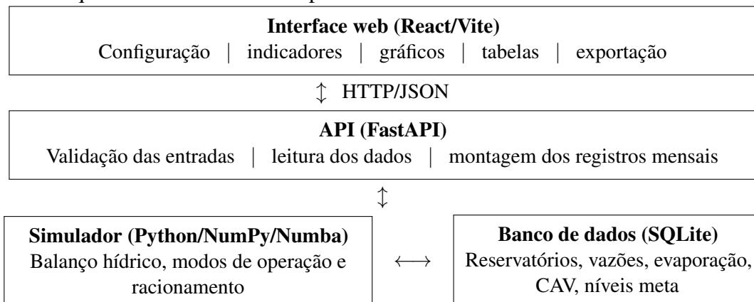
Figura 1 – Arquitetura do sistema de suporte à decisão desenvolvido.
