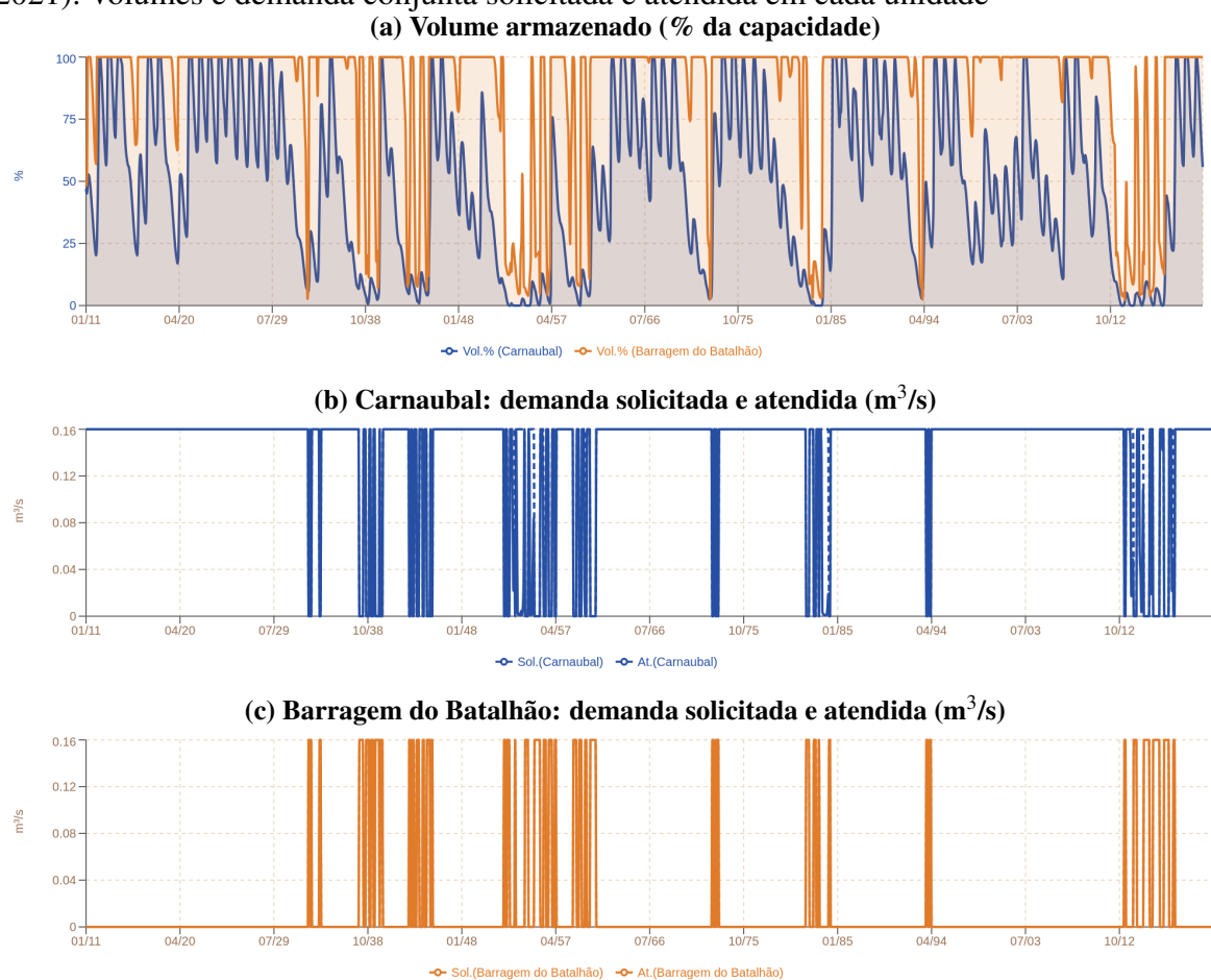
Figura 13: Resultados de Carnaubal–Barragem do Batalhão exportados pelo simulador (1911–2021): volumes e demanda conjunta solicitada e atendida em cada unidade
