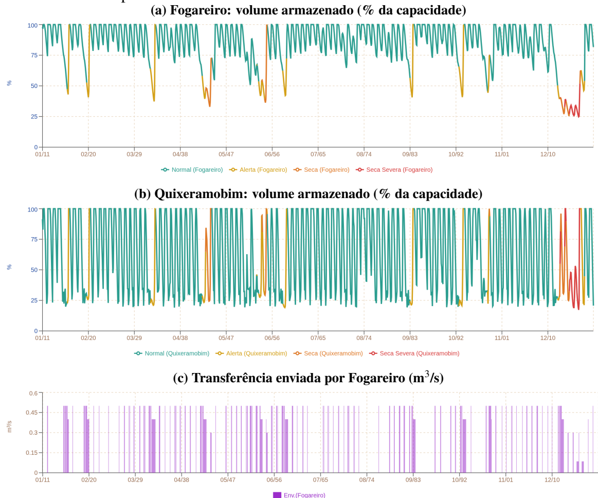
Figura 14 – Resultados de Fogareiro–Quixeramobim exportados pelo simulador (1911–2019): volumes coloridos pelo estado do sistema e vazão transferida.
