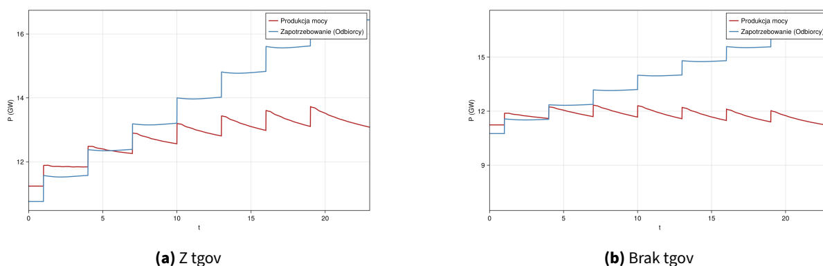
Rysunek 22. Porównanie działania elektrowni z tgov i bez
