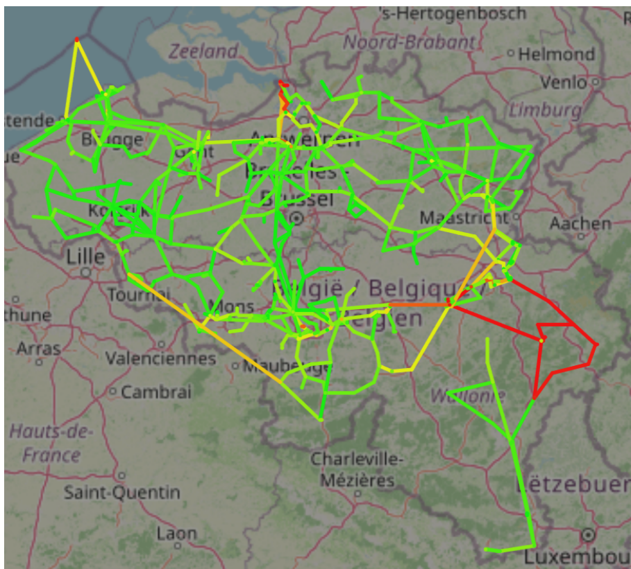
Rysunek 42. Sytuacja po wyłączeniu linii ze zwarcim
