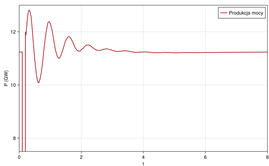
Rysunek 27. Wykres mocy podczas zwarcia
