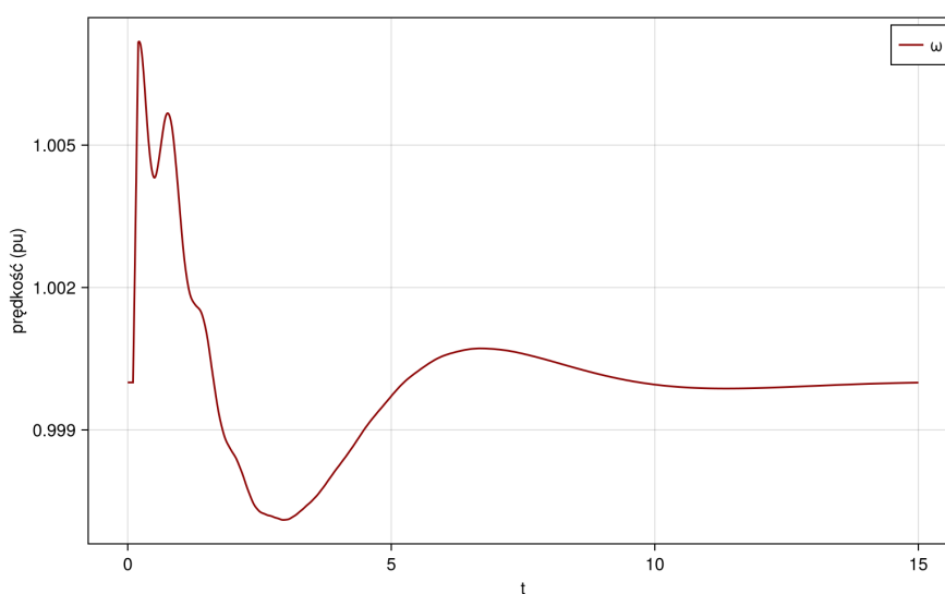
Rysunek 30. Prędkość turbiny
