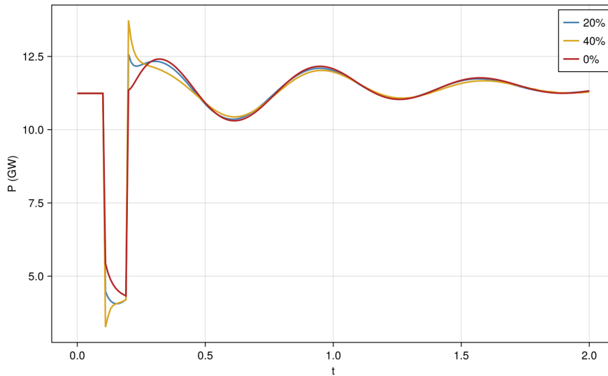
Rysunek 48. Porównanie zachowania dla różnego procentu udziału SimpleGFLDC
