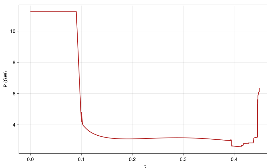
Rysunek 39. Przebieg mocy dla trudnej sytuacji
