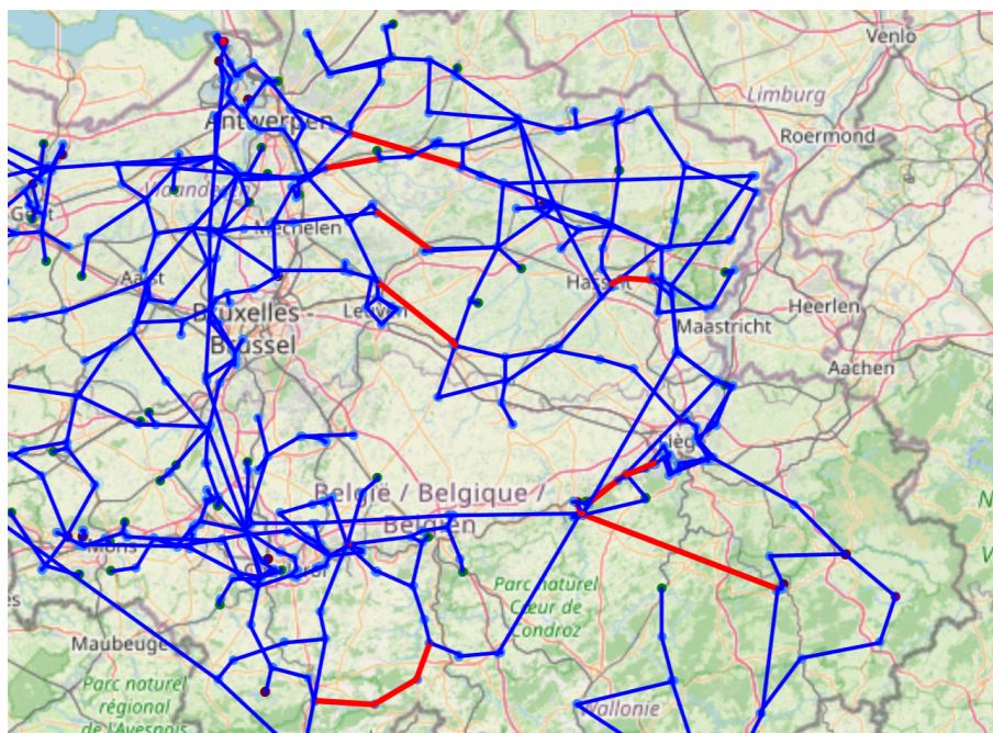
Rysunek 38. Linie wyłączone dla trudnej sytuacji
