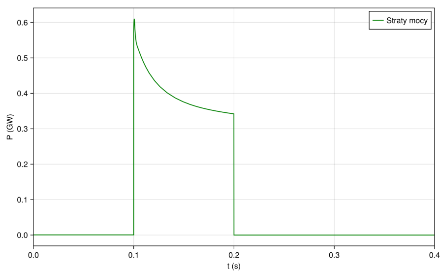
Rysunek 26. Straty mocy na linii ze zwarcie
