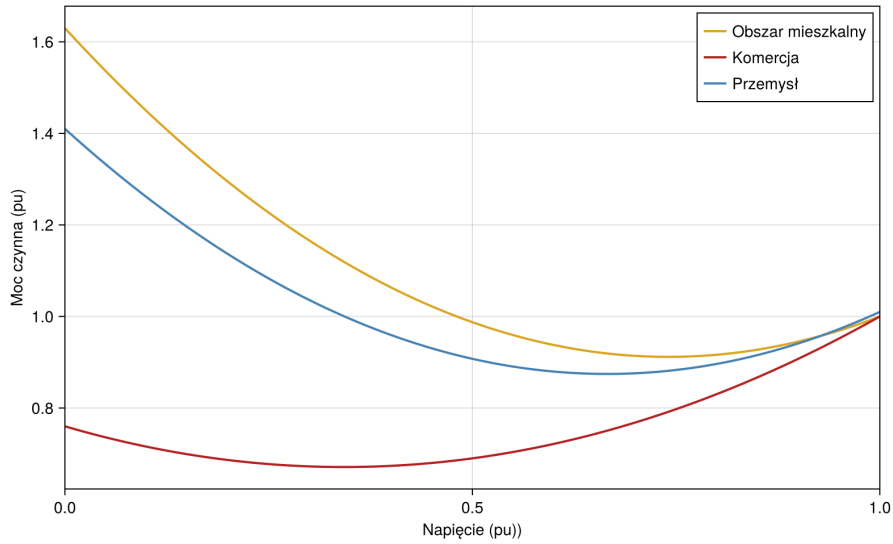
Rysunek 31. Moc czynna dla różnych napięć ZIP_load
