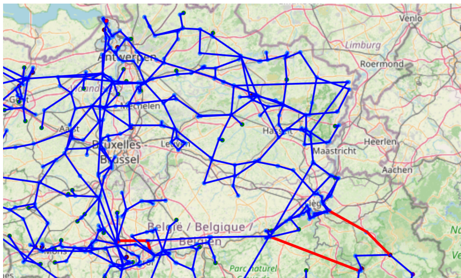
Rysunek 37. Linie wyłączone dla średniej ciężkości sytuacji
