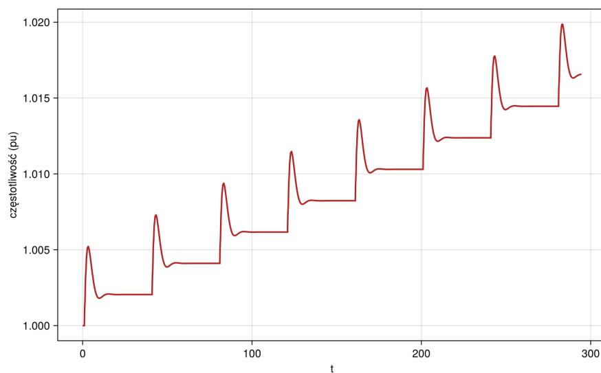
Rysunek 25. Symulacja spadku zapotrzebowania mocy częstotliwość
