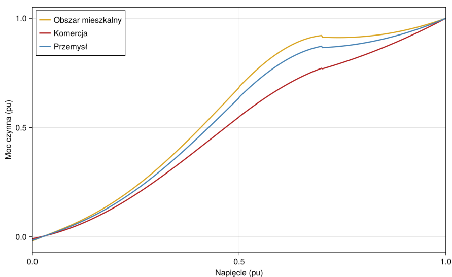
Rysunek 32. Moc czynna dla różnych napięć PSSE_load
