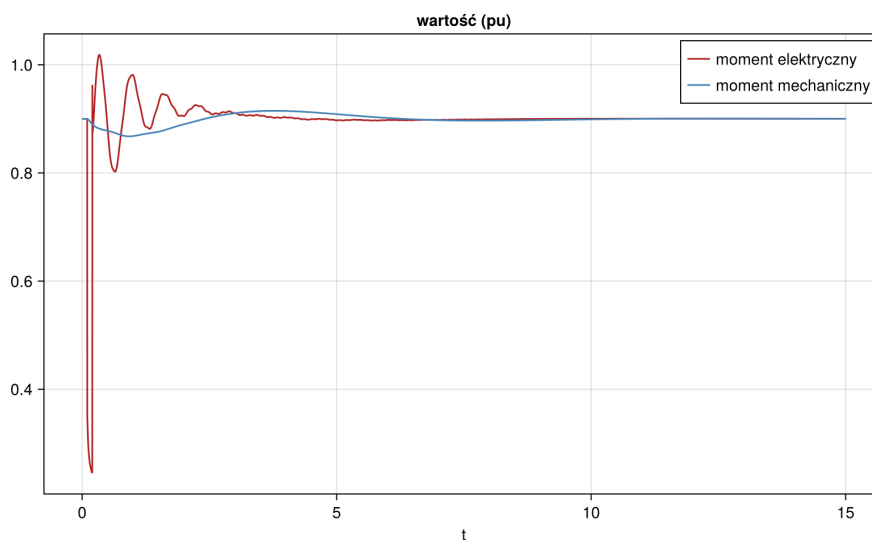
Rysunek 29. Moment mechaniczny
