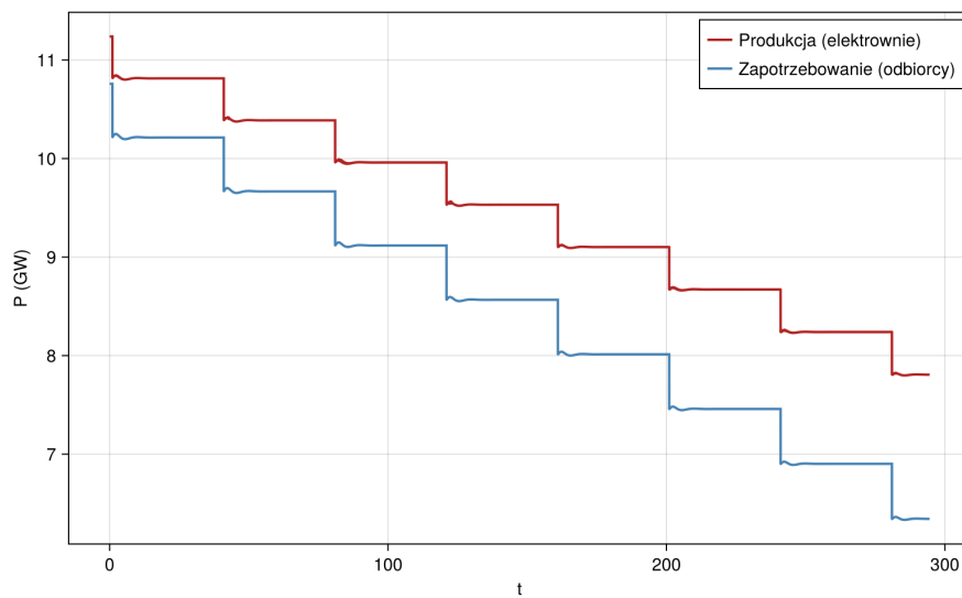
Rysunek 24. Symulacja spadku zapotrzebowania mocy
