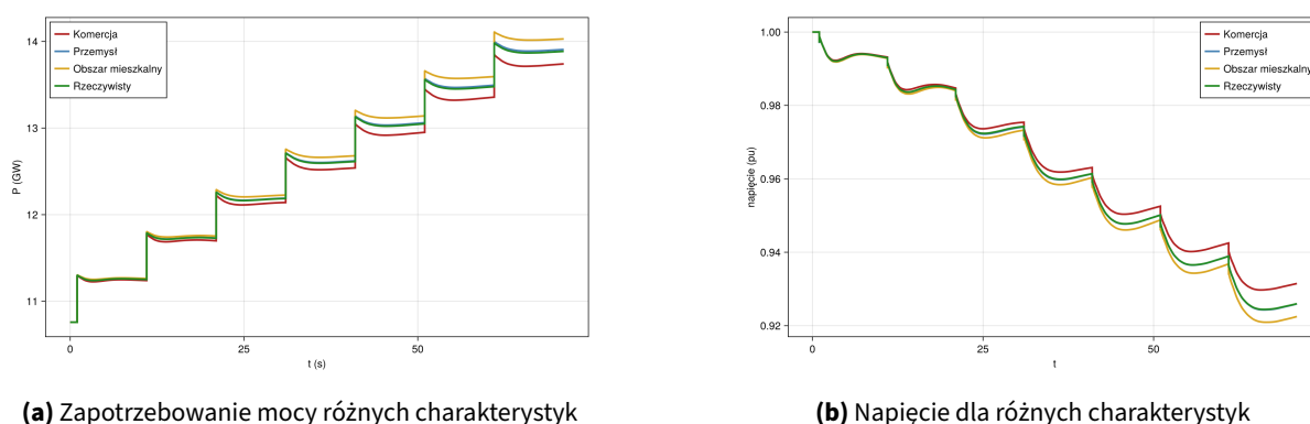
Rysunek 23. Symulacja różnych typów odbiorników
