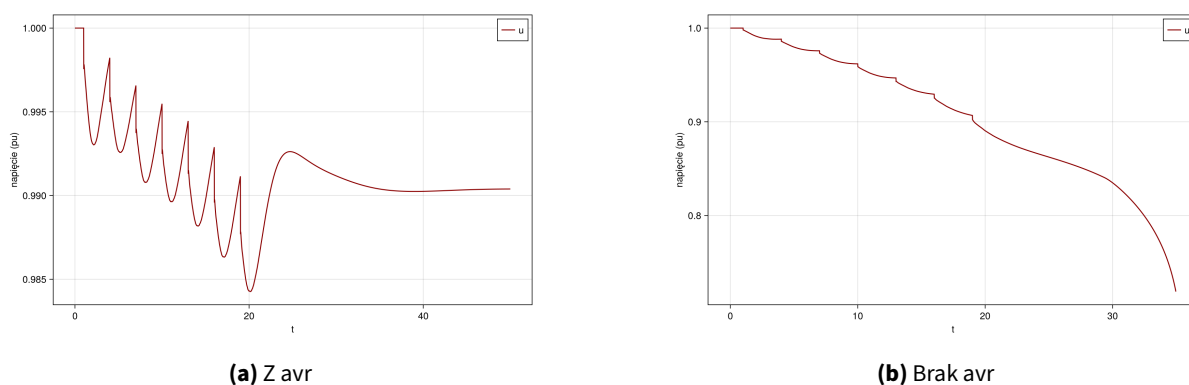
Rysunek 21. Porównanie działania elektrowni z avr i bez
