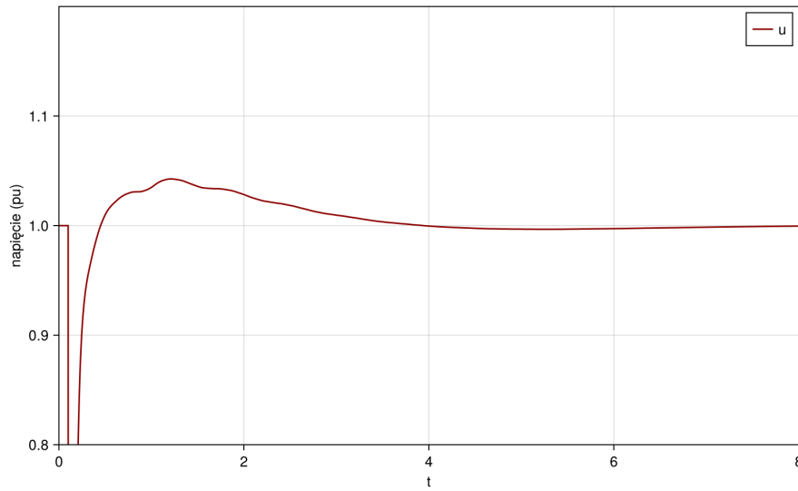
Rysunek 28. Wykres napięcia podczas zwarcia
