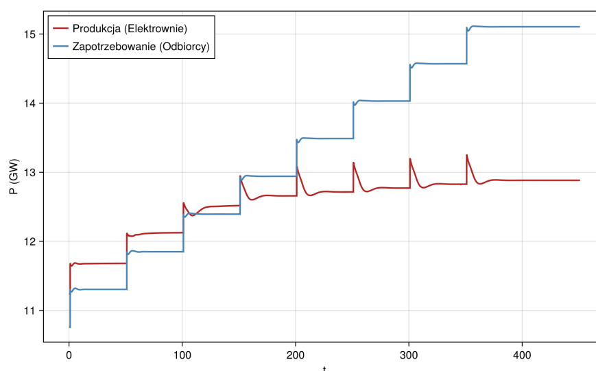
Rysunek 19. Symulacja wzrostu zapotrzebowania mocy
