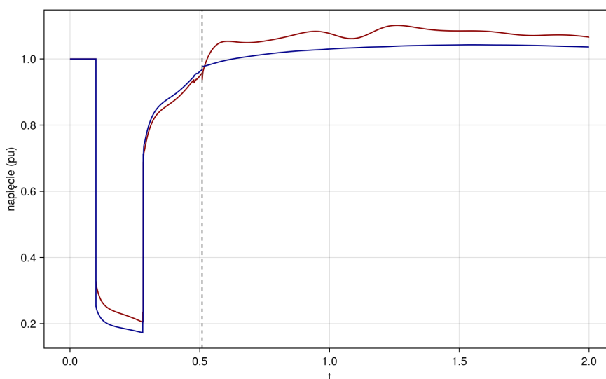
Rysunek 43. Różnica napięcia między odizolowaną siecią, a główną
