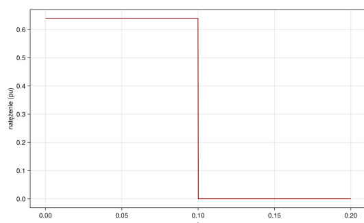
(a) Natężenie na linii wyłączonej
