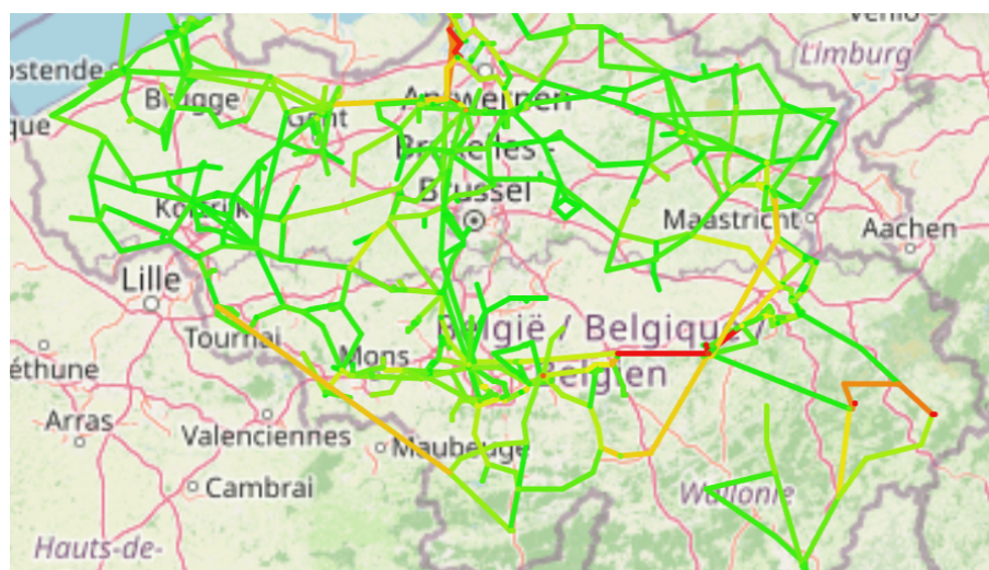
Rysunek 36. Początkowy przepływ mocy
