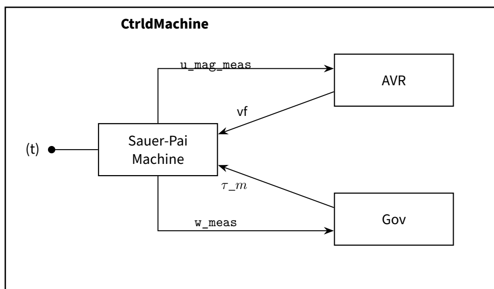
Rysunek 10. Schemat SauerPaiMachine z kontrolowanym napięciem oraz momentem obrotowym.
