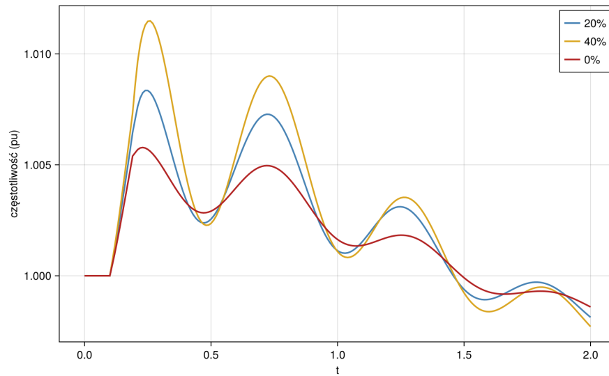
Rysunek 48. Częstotliwość dla różnego procentu udziału SimpleGFLDC
