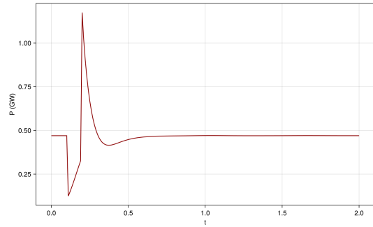
(b) Przebieg mocy dla elektrowni słonecznej
