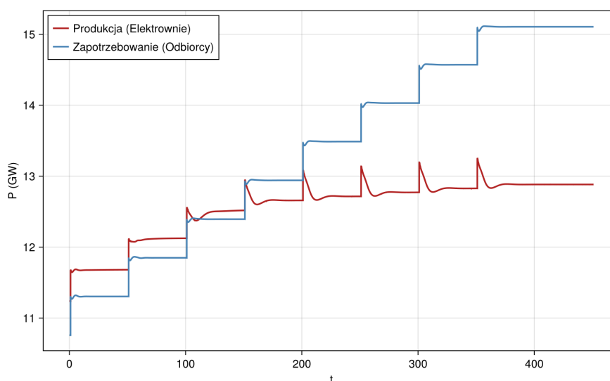
Rysunek 20. Symulacja wzrostu zapotrzebowania mocy
