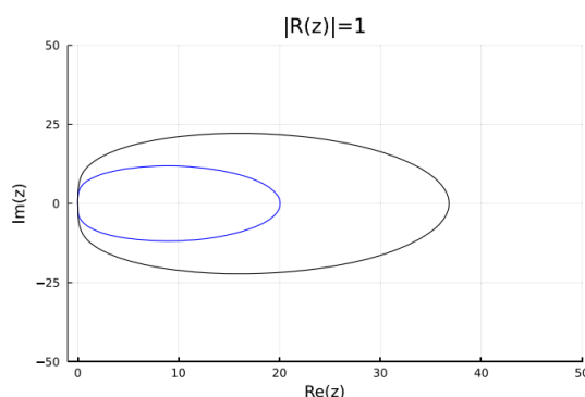
Rysunek 15. Wartości z \in \mathbb{C} z funkcją stabilności |R(z)| = 1 , zaznaczone kolorem czarnym i niebieskim dla jej metody wbudowanej [16]
