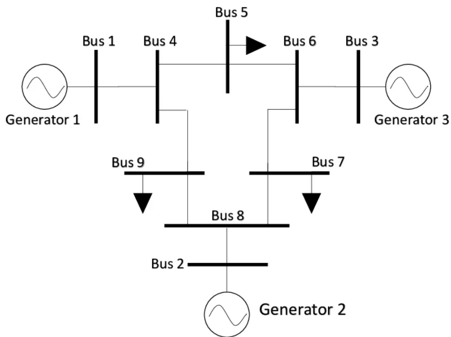
Rysunek 3. IEEE9 [7]
