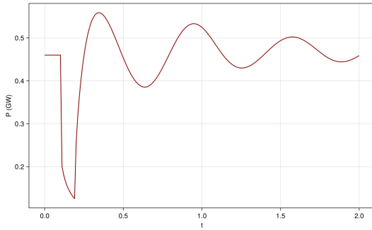
(a) Przebieg mocy dla elektrowni synchronicznej
