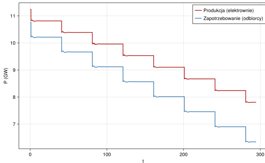
Rysunek 25. Symulacja spadku zapotrzebowania mocy
