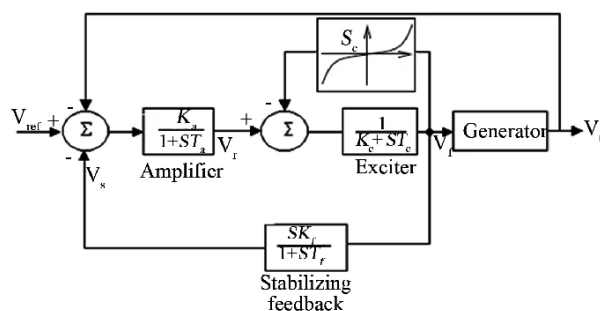
Rysunek 11. AVR [11]
