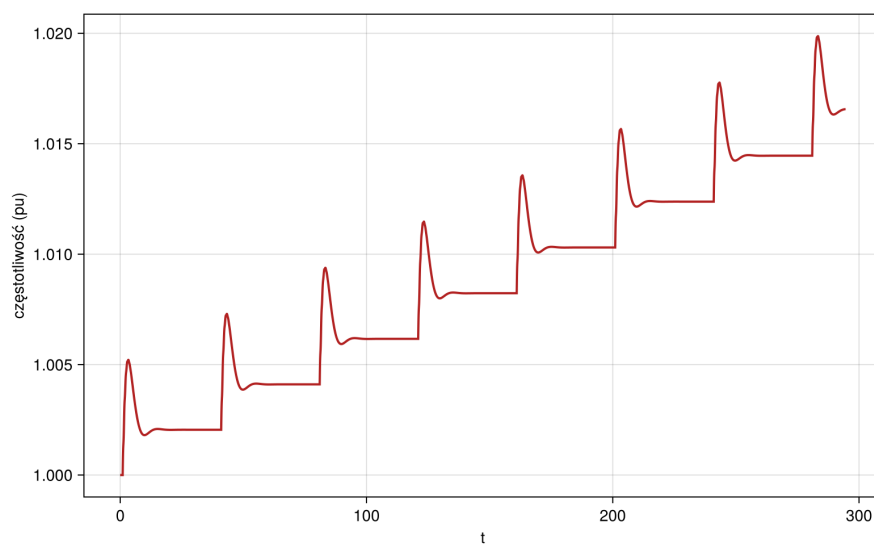
Rysunek 26. Symulacja spadku zapotrzebowania mocy częstotliwość
