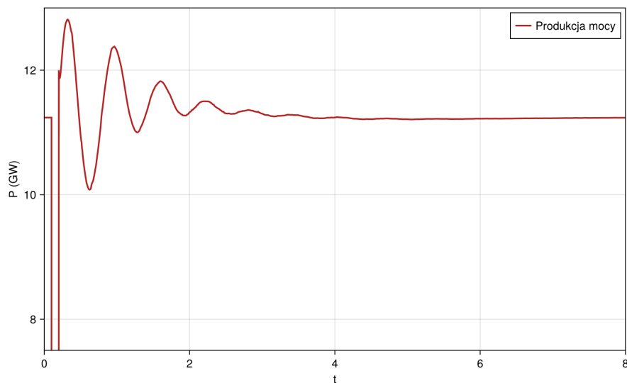
Rysunek 28. Wykres mocy podczas zwarcia
