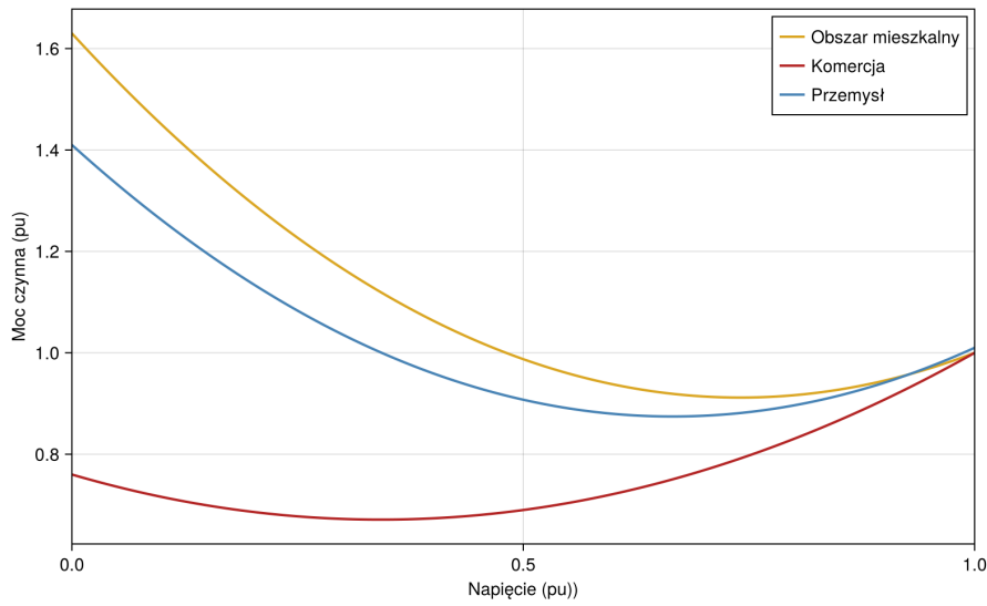
Rysunek 32. Moc czynna dla różnych napięć ZIP_load
