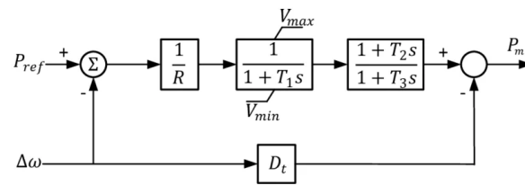
Rysunek 12. TGOV [12]
