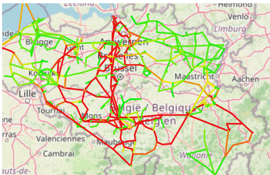
Rysunek 40. Sytuacja po zwarcie
