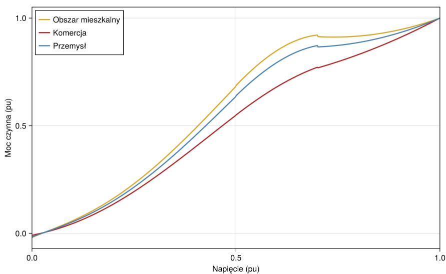
Rysunek 33. Moc czynna dla różnych napięć PSSE_load
