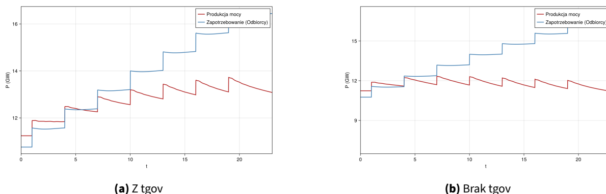
Rysunek 23. Porównanie działania elektrowni z tgov i bez
