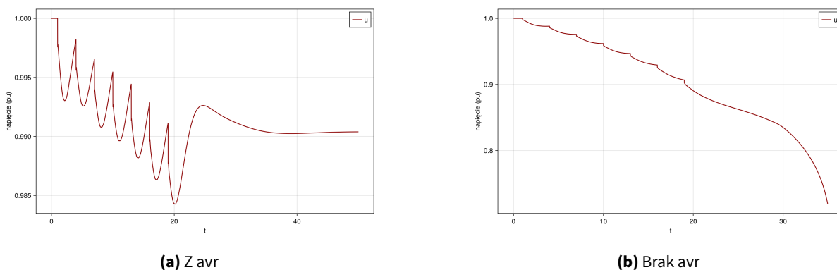
Rysunek 22. Porównanie działania elektrowni z avr i bez
