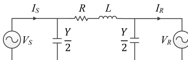
Rysunek 13. pi-line [13]
