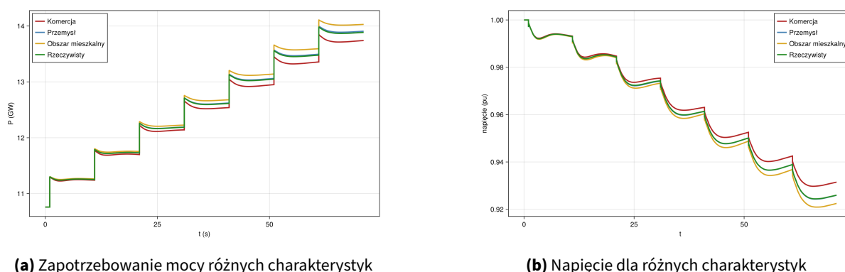
Rysunek 24. Symulacja różnych typów odbiorników
