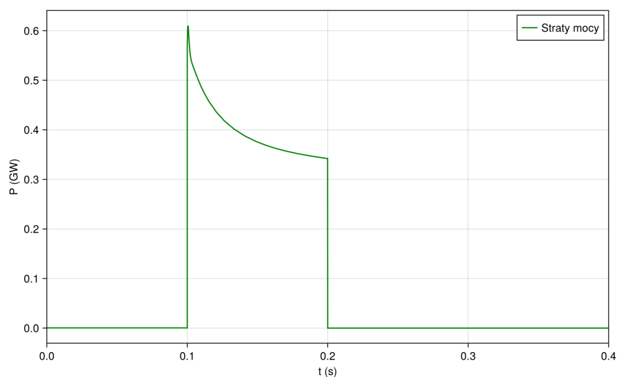
Rysunek 27. Straty mocy na linii ze zwarcie
