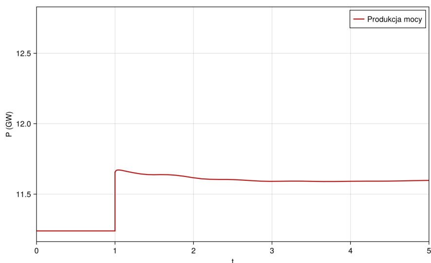
Rysunek 44. Wykres wzrostu mocy
