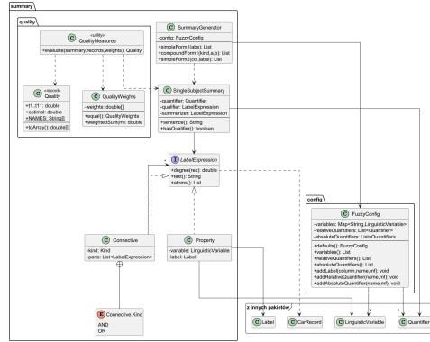
Rysunek 1: Diagram klas pakietów config , summary i summary.quality : konfiguracja zmiennych i kwantyfikatorów ( FuzzyConfig ); wyrażenia summaryzatora/kwalifikatora – interfejs LabelExpression z implementacjami Property (pojedyncza etykieta) i Connective (złożenie spójnikami AND/OR); zdanie jednopodmiotowe i jego generator ( SingleSubjectSummary , SummaryGenerator ); miary jakości T_1 – T_{11} wraz z podsumowaniem optymalnym ( QualityMeasures , rekord Quality , QualityWeights ). Klasy LinguisticVariable , Label , Quantifier i CarRecord pochodzą z innych pakietów (ramka u dołu).
