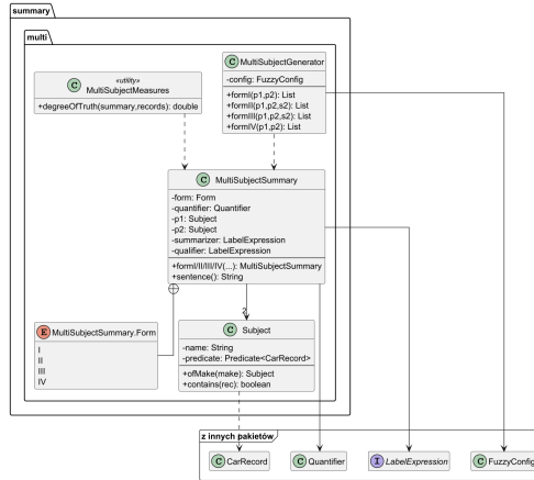
Rysunek 2: Diagram klas pakietu summary.multi – podsumowania wielopodmiotowe w formach I–IV: MultiSubjectSummary (z wyliczeniem Form i fabrykami formI – formIV ), wyróżnianie rozłącznych podmiotów Subject (np. ofMake ), stopień prawdziwości T ( MultiSubjectMeasures ) oraz generator kandydatów ( MultiSubjectGenerator ). Zależności do Quantifier , LabelExpression , FuzzyConfig i CarRecord prowadzą do klas z innych pakietów (ramka u dołu).
