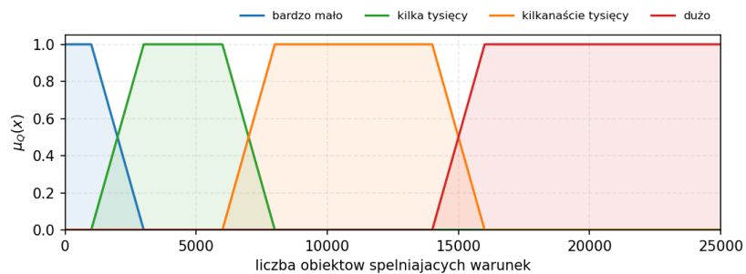
Rysunek 17: Funkcje przynależności czterech kwantyfikatorów bezwzględnych zdefiniowanych na przestrzeni X_Q^{abs} = [0, 25\,000] . Argumentem jest liczba obiektów spełniających warunek.
