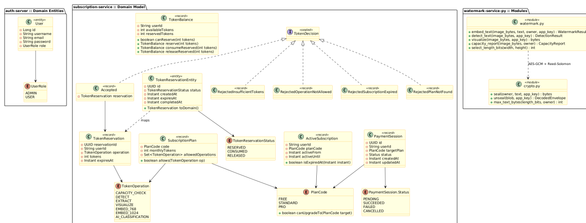
Rysunek 4: Diagram klas domenowych systemu StegoCloud
