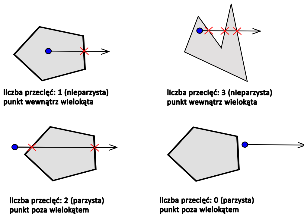
Rysunek 3.3: Wizualna reprezentacja algorytmu rzucania promienia
