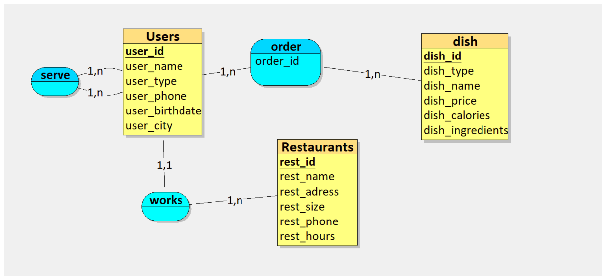
ER diagramm
