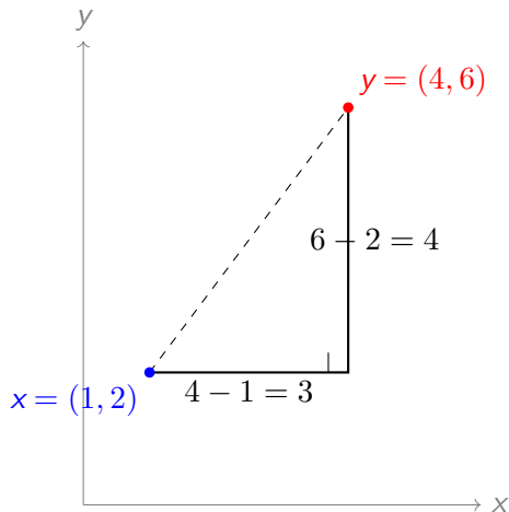
Figura 1: Representação da distância de Manhattan entre os pontos x e y
