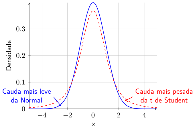
Figura 6: Comparação entre a distribuição Normal padrão e a t de Student com \nu = 3 . A t possui caudas mais pesadas, o que a torna mais robusta a outliers.
