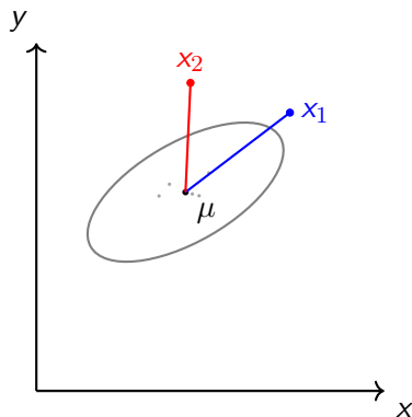
Figura 3: Representação simplificada da distância de Mahalanobis
