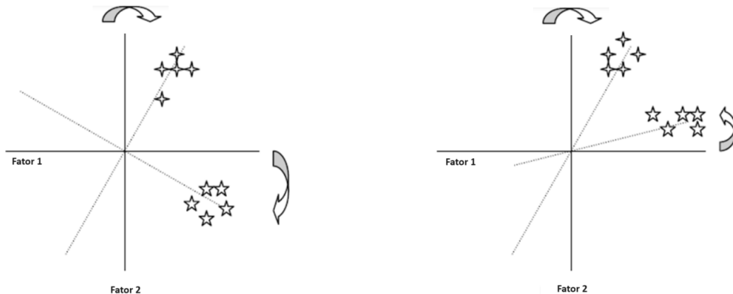
Figura 7: Representação gráfica da rotação ortogonal de fatores.
