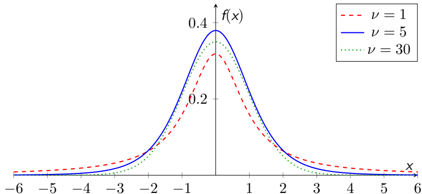
Figura 5: Distribuições t de Student com diferentes graus de liberdade \nu .
