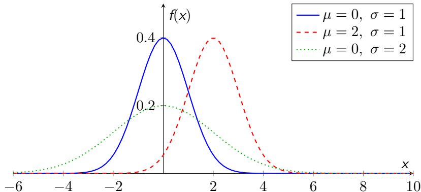
Figura 4: Três distribuições normais com diferentes médias e desvios-padrão.
