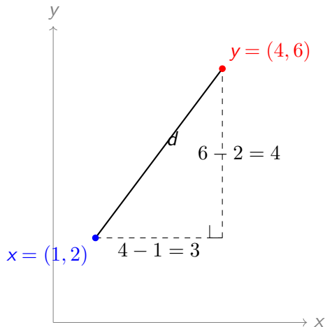
Figura 2: Representação geométrica da distância euclidiana entre os pontos x e y
