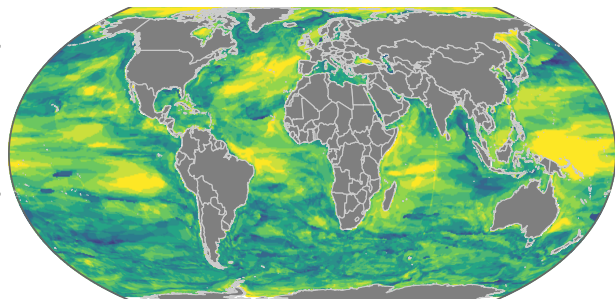
Total Zooplankton
