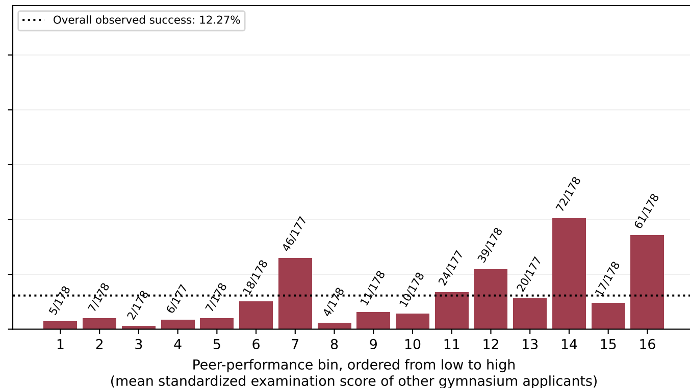
Quantile bins (16)
