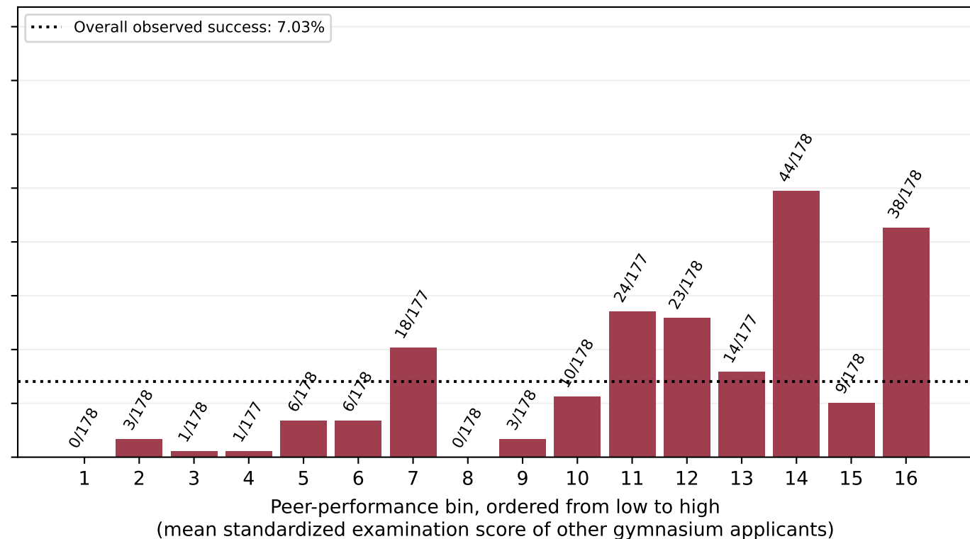
Quantile bins (16)
