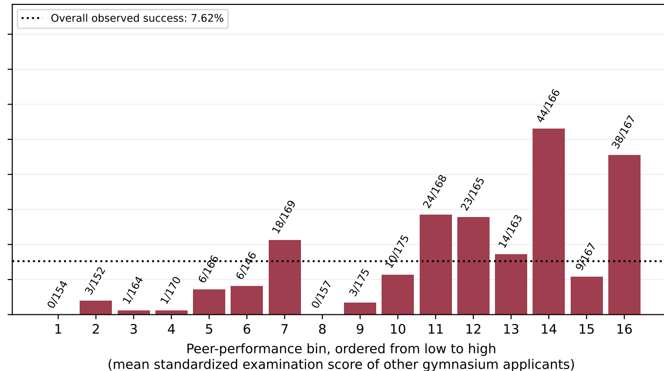
Quantile bins (16)
