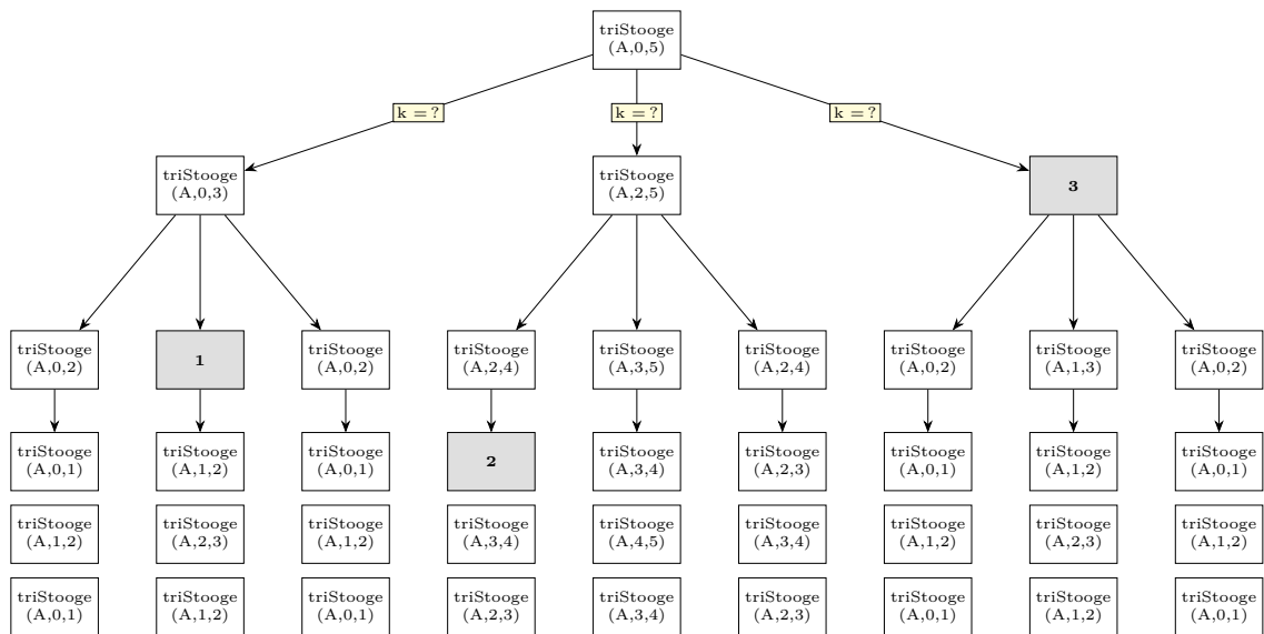
Arbre des appels récursifs pour triStooge(A, 0, 5) (au dernier niveau, les trois appels issus d'un même nœud sont empilés verticalement).
