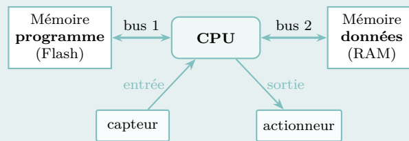
architecture de Harvard : deux mémoires, deux bus
