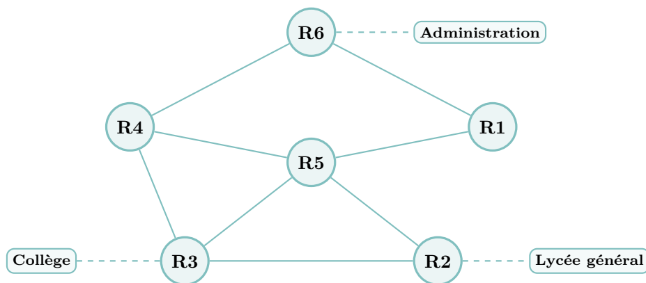
Figure 1 : les routeurs de l'établissement (en pointillés : le routeur qui dessert un secteur)
