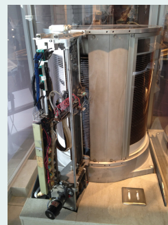
Le mécanisme du disque IBM 350 (1956)
