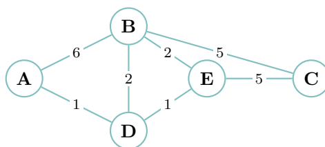
Le graphe pondéré G du projet ( poids = distances ).
