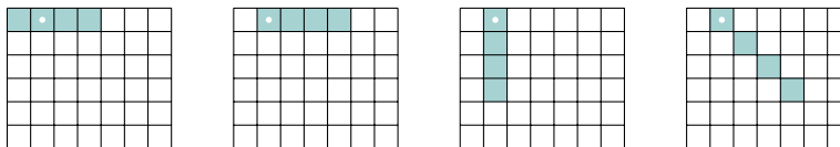
Figure 2. Les alignements contenant la case (0, 1) (marquée d'un point blanc).
