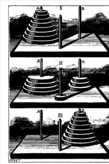
Les tours de Hanoï (É. Lucas, 1883)
