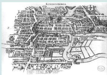
Königsberg et ses ponts (gravure de 1652)
