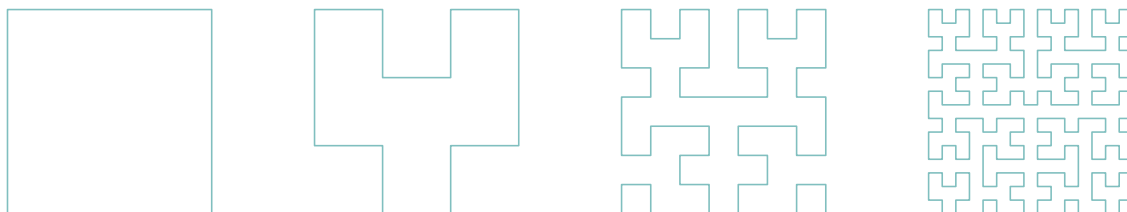
La courbe de Hilbert, aux ordres n = 1, 2, 3 puis 4.
