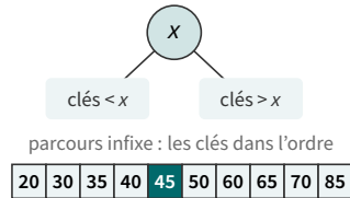
Arbre binaire de recherche
