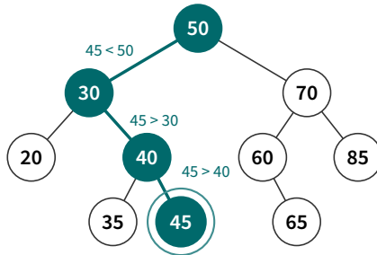
Arbre binaire de recherche
