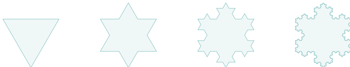
Le flocon de Koch, aux étapes n = 0, 1, 2 puis 4.
