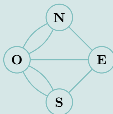
Le graphe d'Euler
