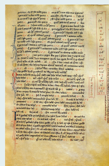
Le problème des lapins dans le Liber abbaci
