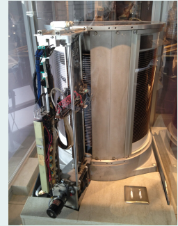
Le mécanisme du disque IBM 350 (1956)
