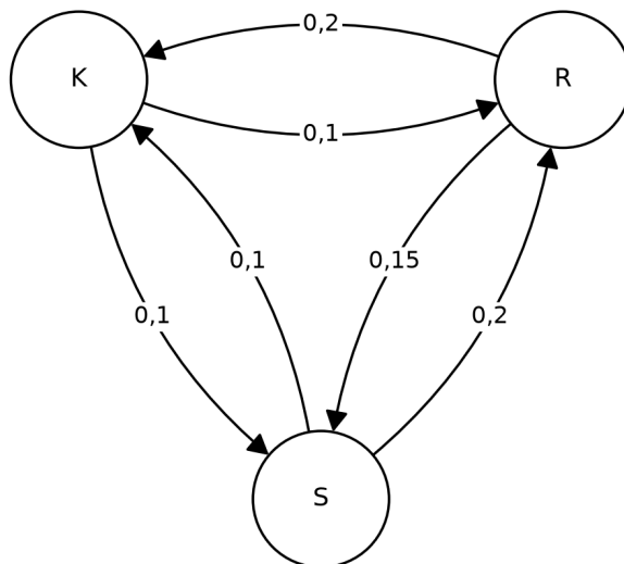
Figure 4: Alt-Text: Übergangsgraph der Anbieter K, R und S
