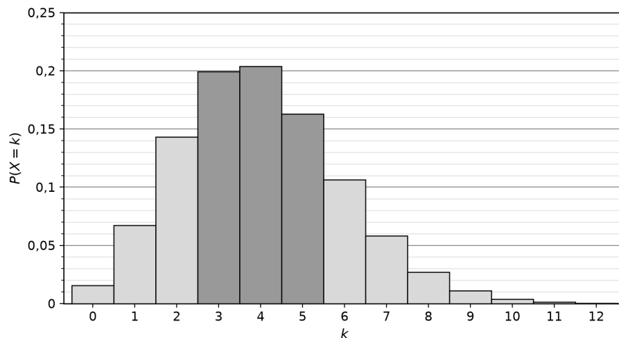
Figure 3: Alt-Text: Histogramm der Wahrscheinlichkeitsverteilung von X ; die Balken des Ereignisses E_3 sind dunkel hervorgehoben
