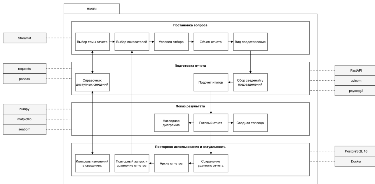
Рис. 8: Модульная архитектура бизнес процессов
