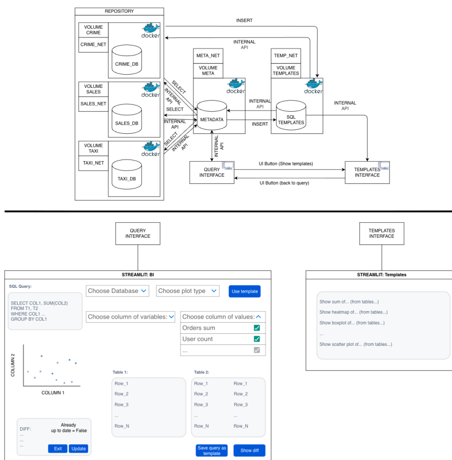
Рис. 6: Архитектура программы
