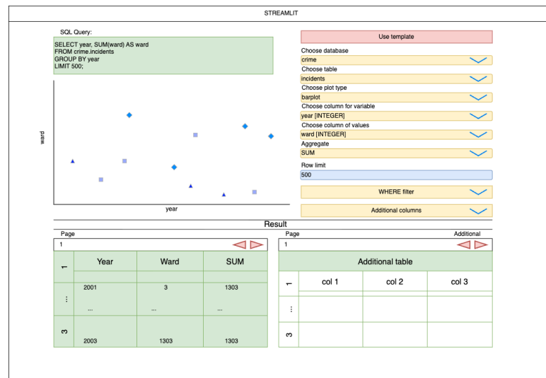
Рис. 13: Шаблон интерфейса
