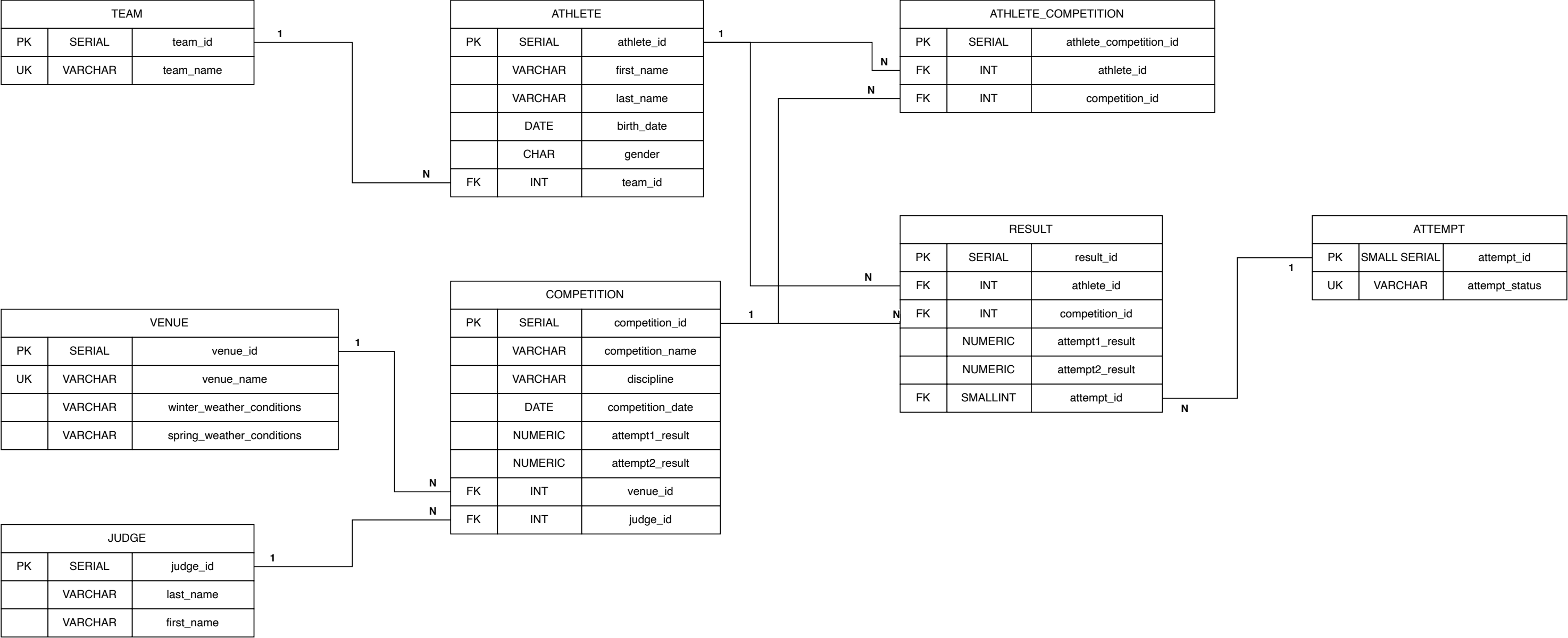
Рис. 2: Архитектура базы данных горнолыжных соревнований
