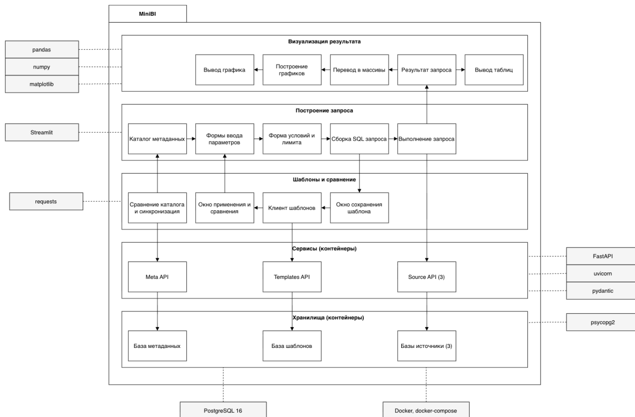
Рис. 7: Модульная архитектура программы
