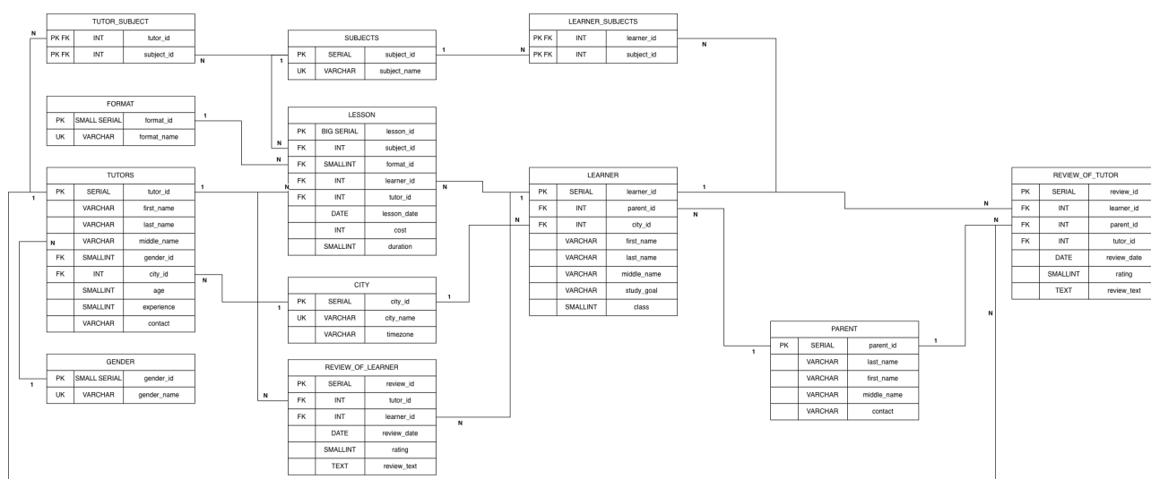
Рис. 2: Архитектура базы данных учета репетиторов
