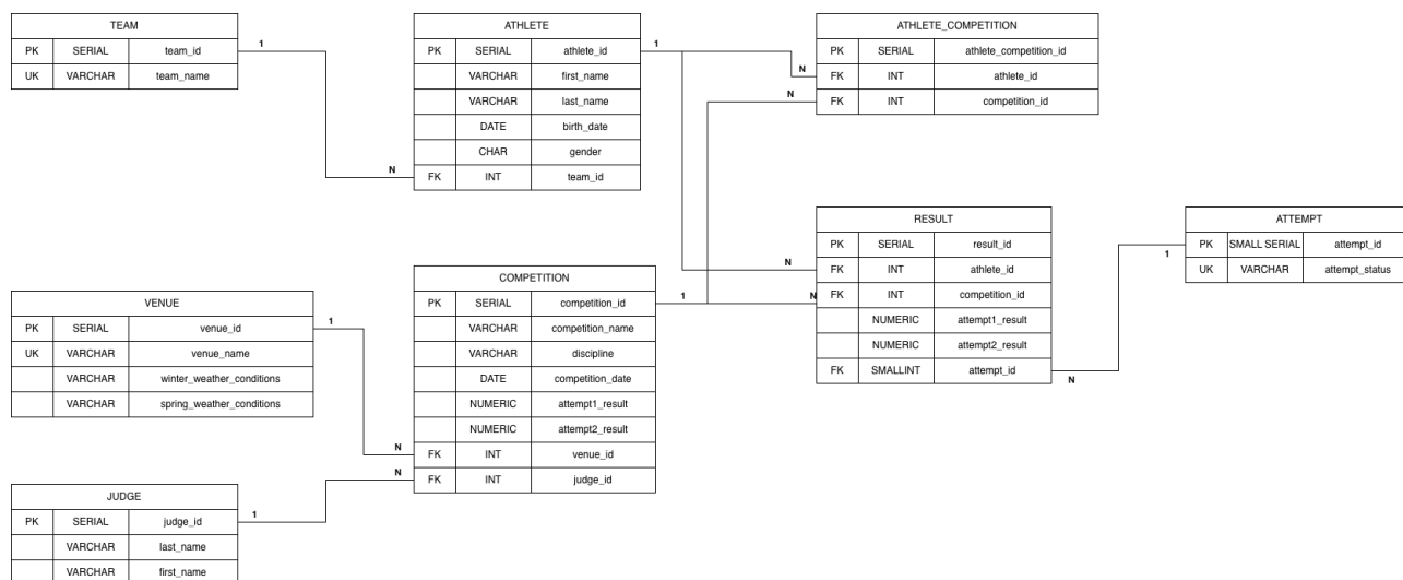
Рис. 3: Архитектура базы данных горнолыжных соревнований
