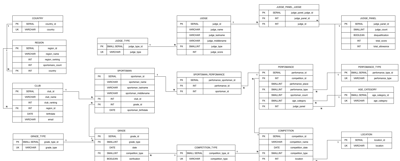
Рис. 4: Архитектура базы данных спортсменов и соревнований в чирлидинге
