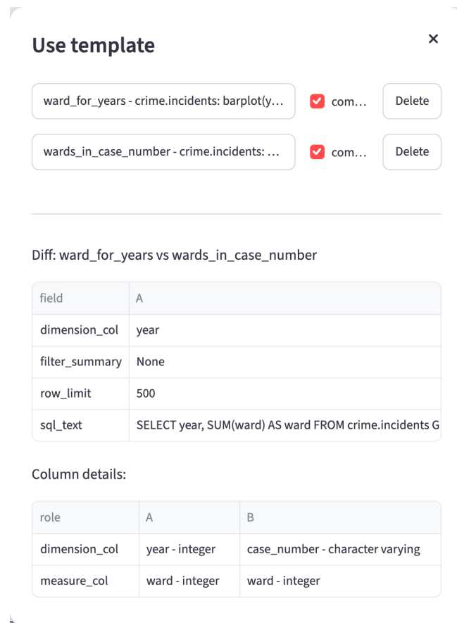
Рис. 18: Итоговый интерфейс сравнения шаблонов
