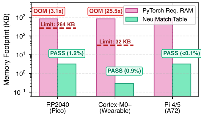
(d) Microcontroller Feasibility
