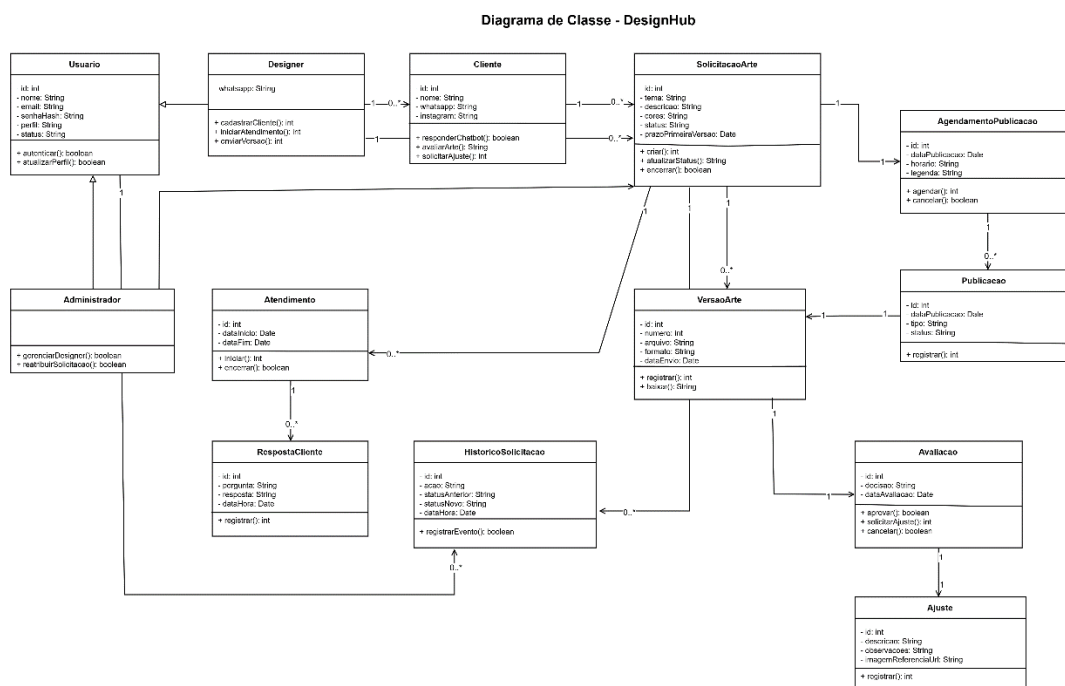
FIGURA 33 – Diagrama de Classe
