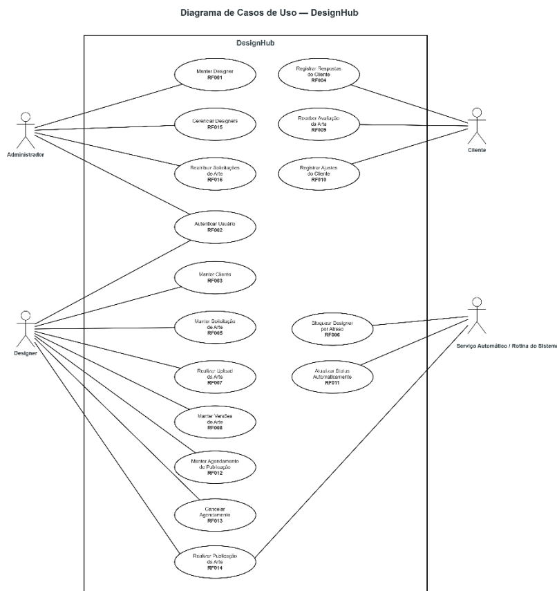
FIGURA 30 – Diagrama de caso de uso
