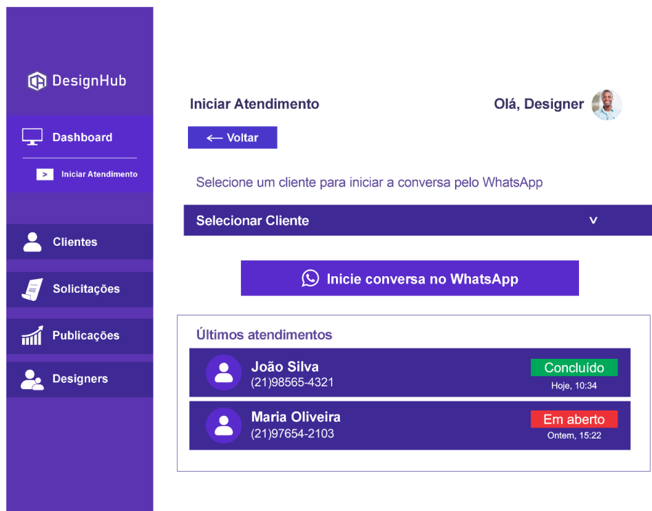
FIGURA 8 – Iniciar Atendimento
