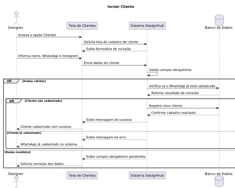
FIGURA 31 – Diagrama de sequência (Incluir cliente)
